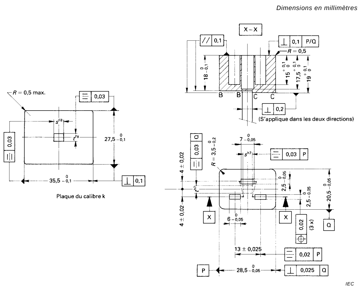
Figure 20 – Calibre "ENTRE" pour socles de connecteurs selon les feuilles de norme C20 et C24
