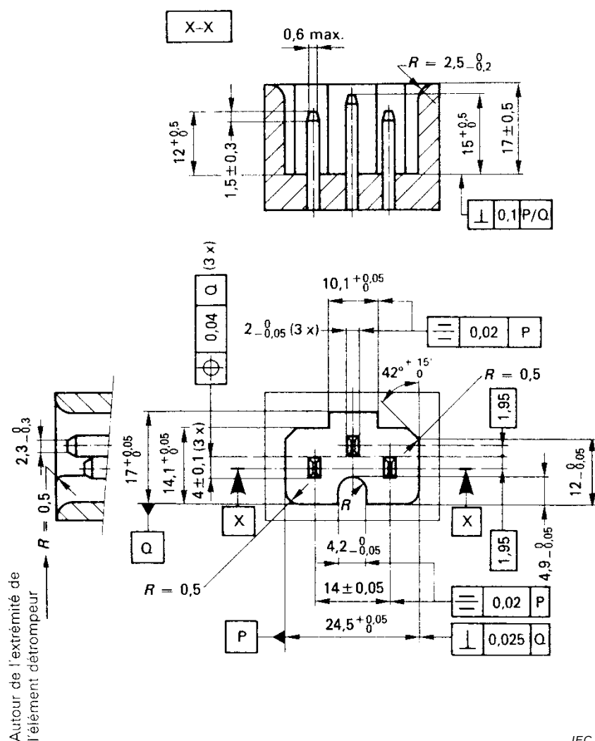
Figure 24 – Calibre "N'ENTRE PAS" pour prises mobiles selon les feuilles de norme C13, C15 et C17
