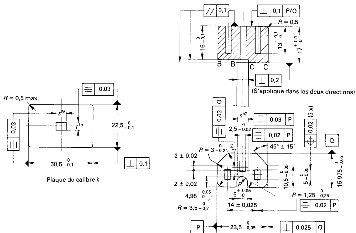
Figure 16 – Calibre "ENTRE" pour socles de connecteurs selon les feuilles de norme C14, C16 et C18
