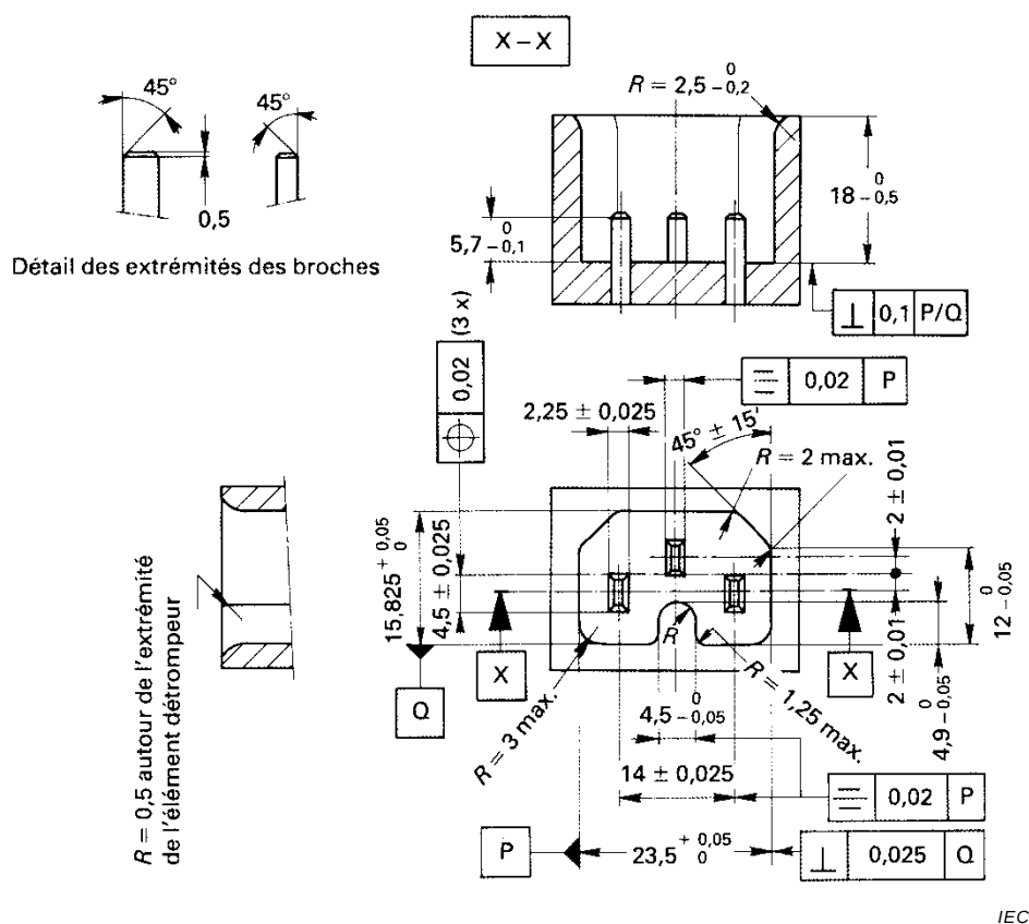
Figure 17 – Calibre "ENTRE" pour prises mobiles selon la feuille de norme C15
