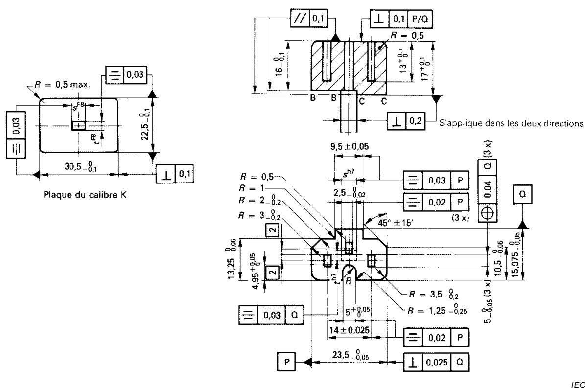
Figure 26 – Calibre "ENTRE" pour socles de connecteurs selon la feuille de norme C16A
