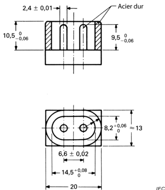
Figure 2 – Calibre "ENTRE" pour prises mobiles selon la feuille de norme C1
