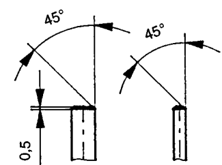
Détail des extrémités des broches
