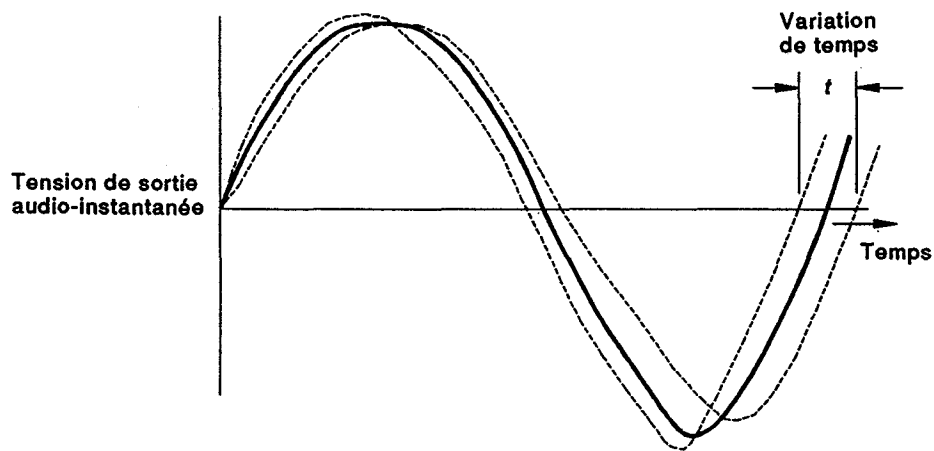
Figure 6 - Mesure de la déviation maximale de fréquence provoquée par une modulation de fréquence résiduelle, une vibration ou un choc (voir 2.15.1)
