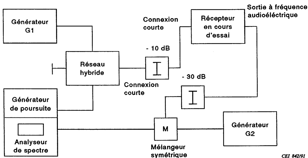
Figure 2 - Montage de mesure de la sélectivité avec une fréquence pilote (voir 2.7.4)
