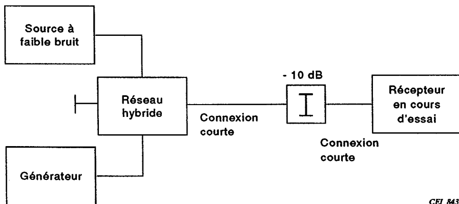
Figure 3 - Montage de mesure du niveau d'interception de 3 e ordre (voir 2.8.1)
