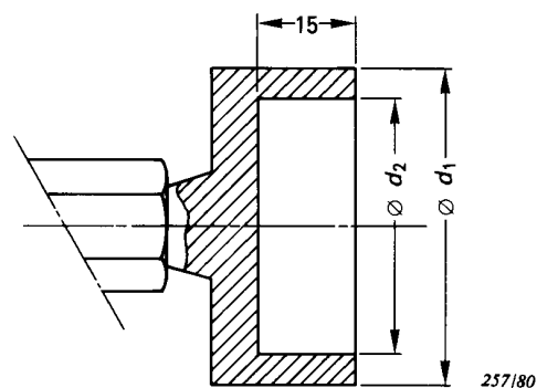
CALIBRE B POUR VÉRIFIER \varnothing d_2 GAUGE B FOR CHECKING \varnothing d_2
