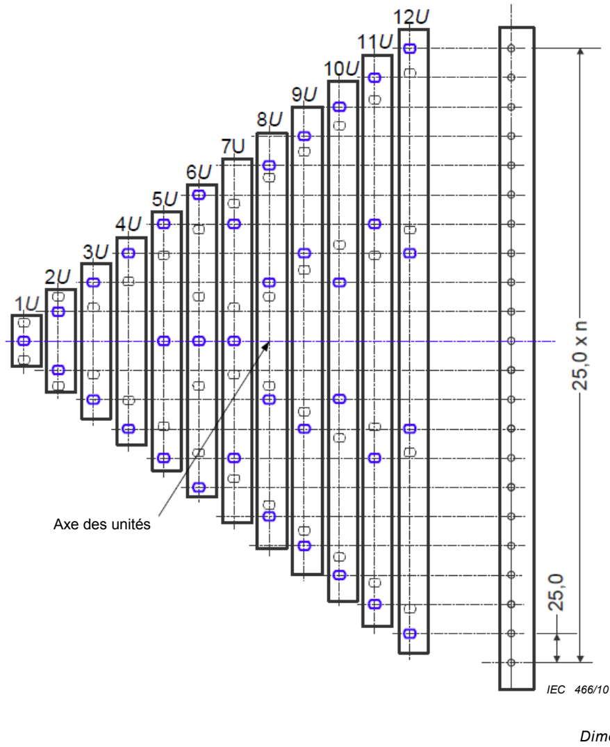
Figure 4 – Dispositions des trous de montage sur les brides, installation de montage par rapport aux axes des bacs ou des châssis de 19 pouces
