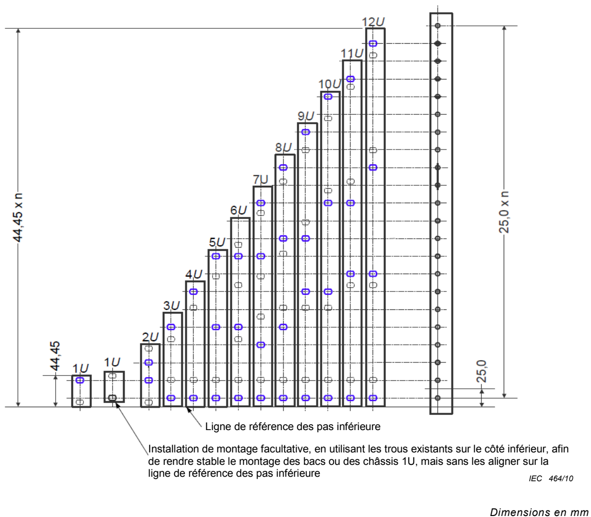
Figure 2 – Dispositions des trous de montage sur les brides, installation de montage par rapport aux lignes de référence des pas inférieures des bacs ou des châssis de 19 pouces
