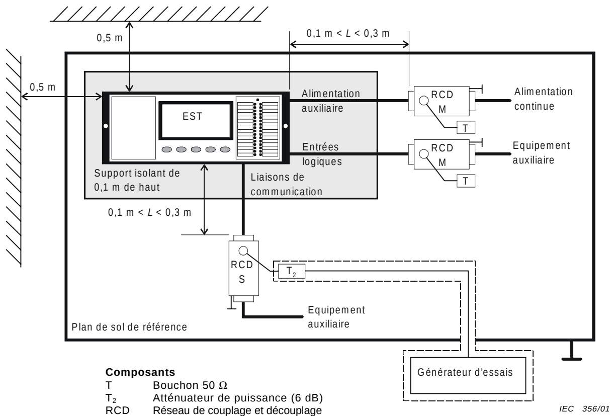
Figure 2 – Exemple de montage d'essais pour équipement seul utilisant des RCD
