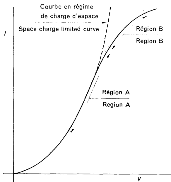
FIG. 1. — Courbe du courant d'émission en fonction de la tension. Emission current-voltage curve.
