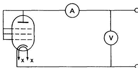
FIG. 2. — Disposition du circuit de mesure du courant d'émission par la méthode 1A ou 1B. Circuit arrangement for measurement of emission current by Method 1A or 1B.
