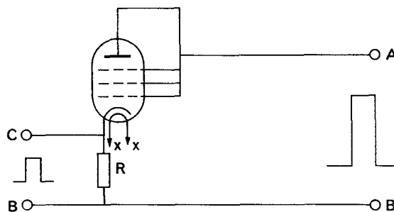
FIG. 3. — Branchement pour mesurer le courant d'émission par la méthode 2A. Connections for measurement of emission current by Method 2A.
