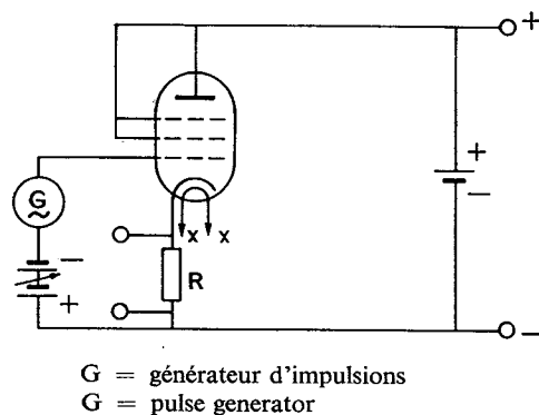
FIG. 4. — Branchement pour mesurer le courant d'émission par la méthode 2B. Connections for measurement of emission current by Method 2B.
