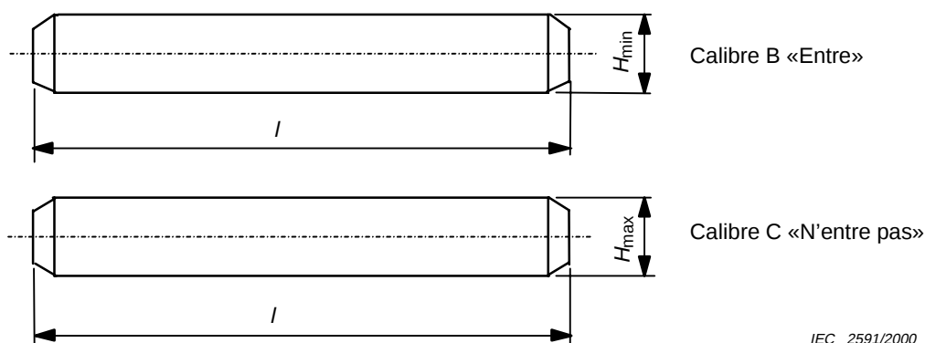
Figure C.2 – Dimensions des calibres B et C
