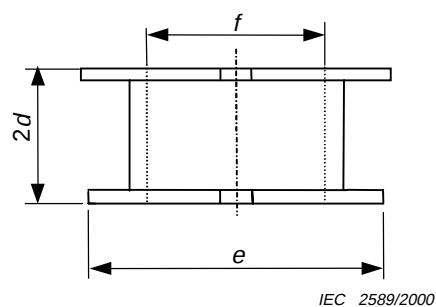
Figure 3 – Dimensions principales des carcasses
