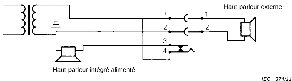
Figure C.1 – Fiche 60130-9 IEC-05 insérée en position A
