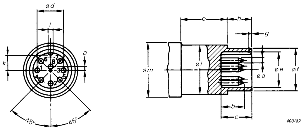
Figure 21 – Fiche 60130-9 IEC-20
