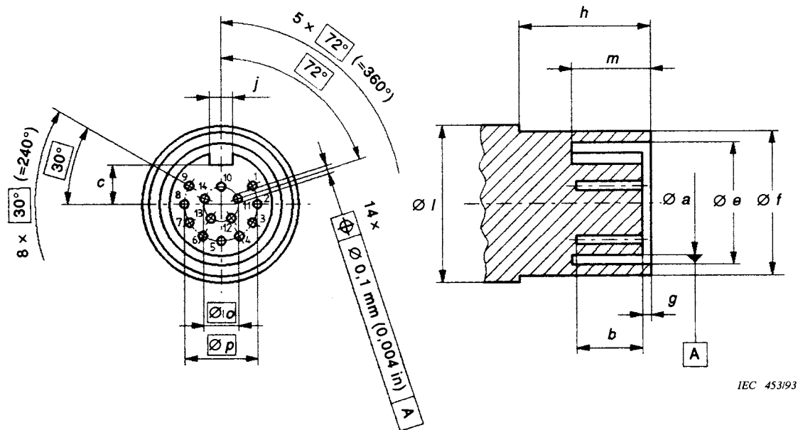
Figure 24 – Fiche 60130-9 IEC-27
