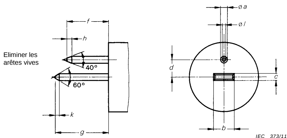
Figure 34 – Calibre pour les essais de tenue en tension et de résistance de contact des connecteurs 60130-9 IEC-08
