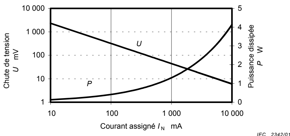
Figure 1 – Exemple de puissance dissipée P et chute de tension U selon le courant assigné I_N
