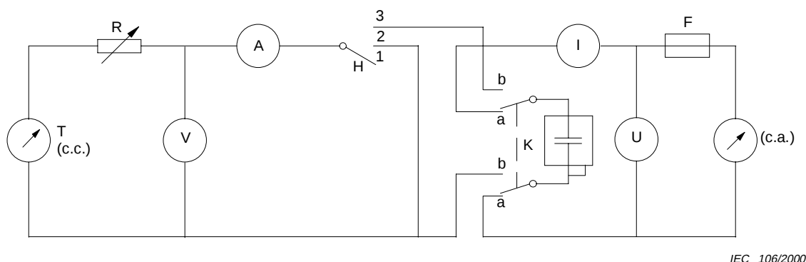
Figure 1 – Schéma pour effectuer l'essai de destruction
