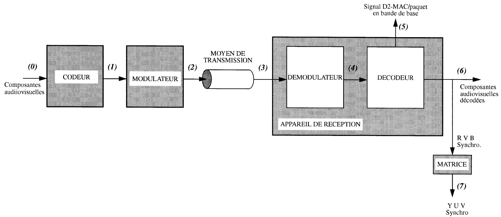
Figure 1 – Schéma de principe de la chaîne de référence fictive
