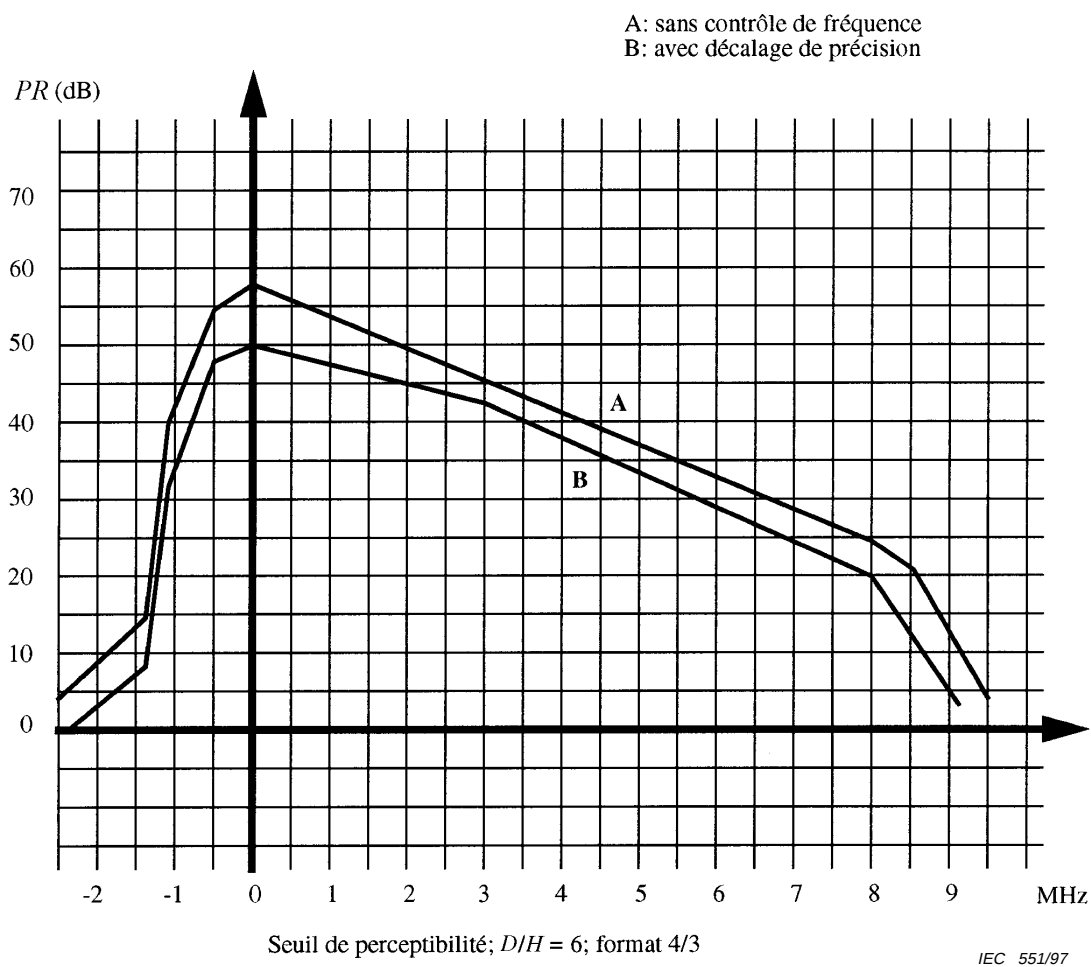
Figure B.4 – Exemple de rapport de protection contre les interférences en MA-BLR
