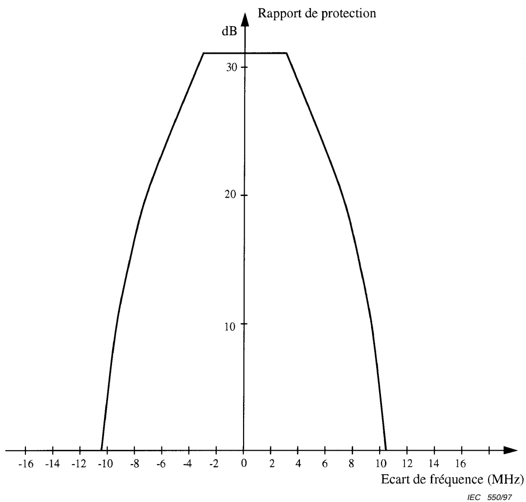
Figure B.3 – Exemple de rapport de protection contre les interférences en FM
