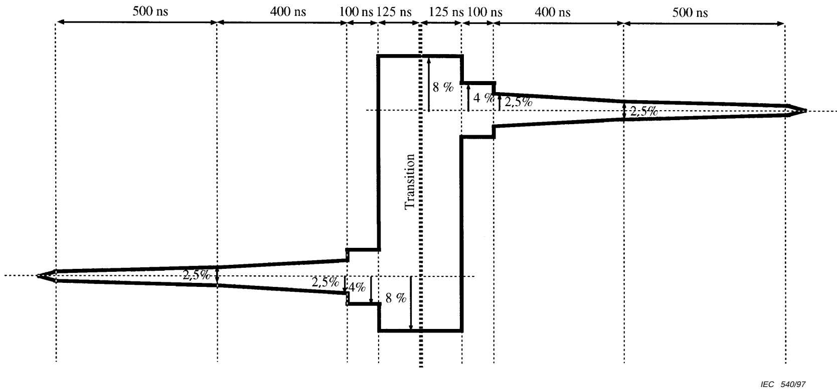
Figure 10 – Exemple de gabarit pour la réponse à un échelon formé
