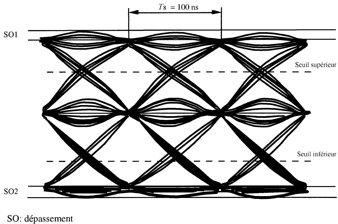
Figure 2 – Diagramme de l'oeil pour le signal duobinaire
