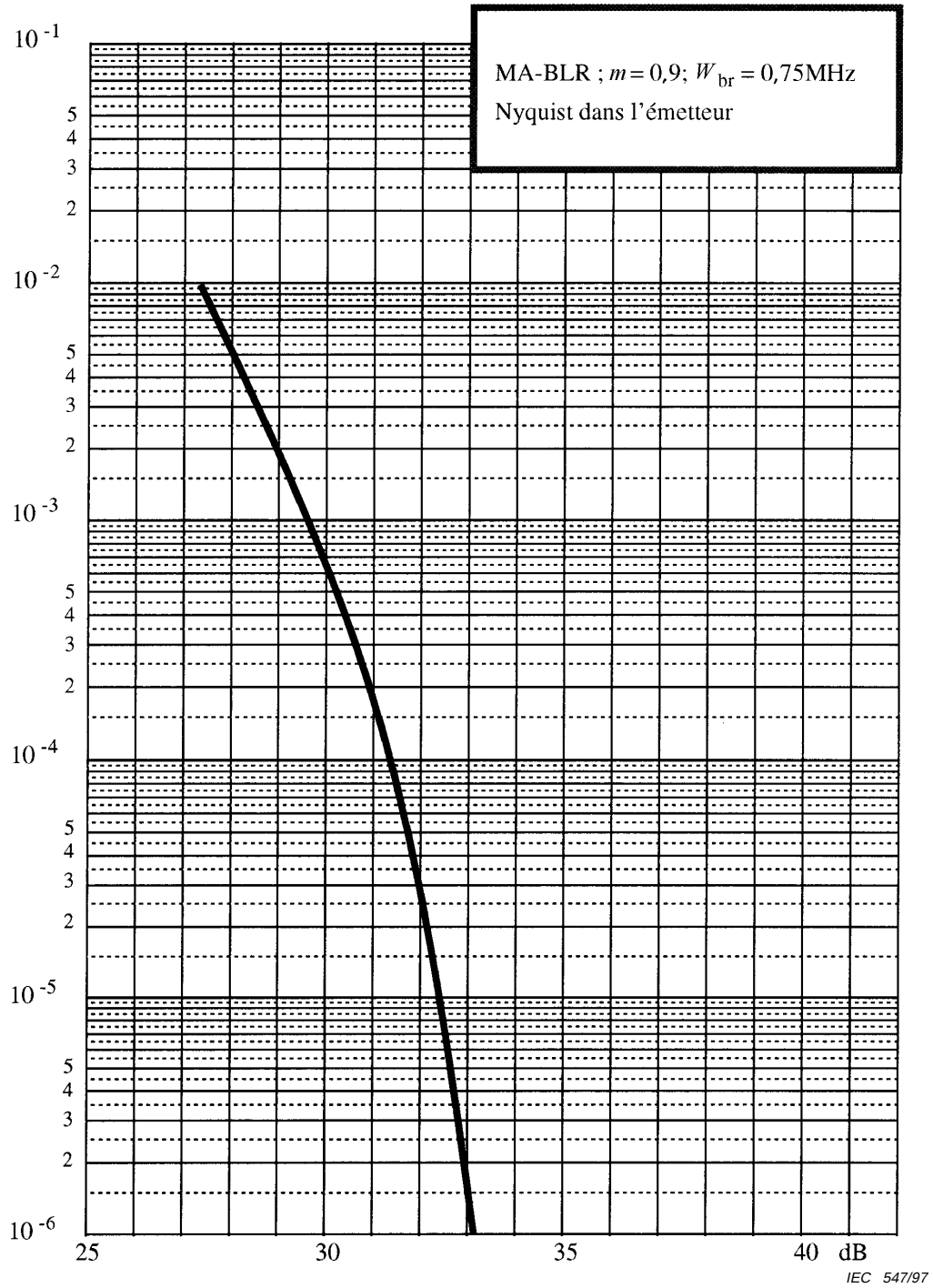
Figure A.5 – Taux d'erreur en fonction du C/N (largeur de bande de mesure de bruit W = 1\text{ MHz} )
