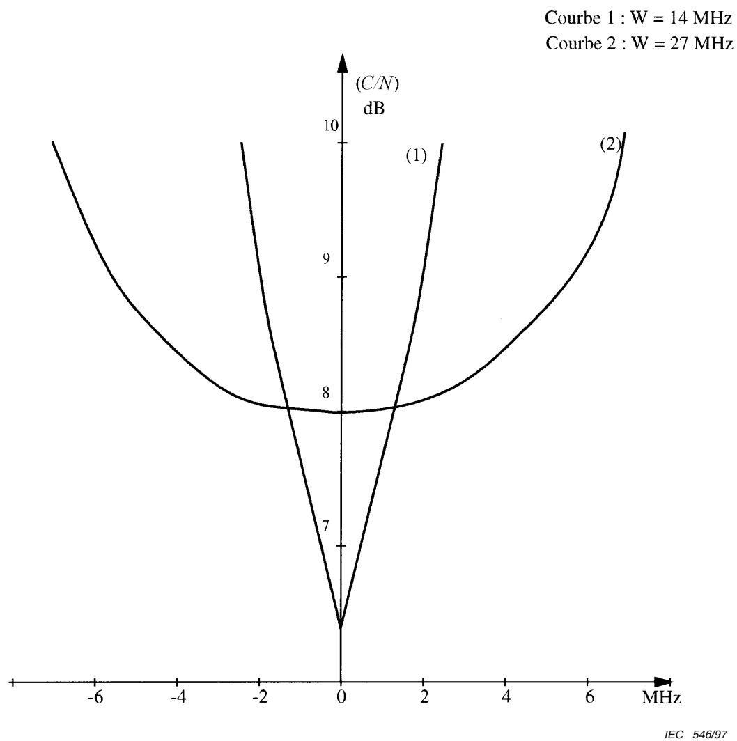
Figure A.4 – Exemple de dégradation équivalente pour un décalage en fréquence de la porteuse à 10^{-3} de taux d'erreur
