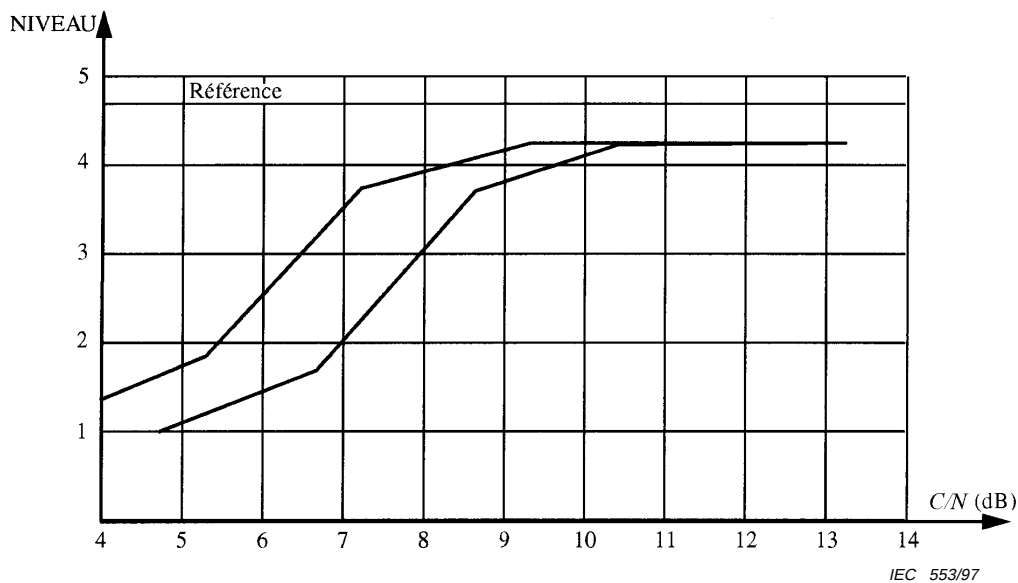
Figure B.5 – Résultat de mesure sur la qualité du signal d'image en fonction du C/N en 27 MHz de largeur de bande
