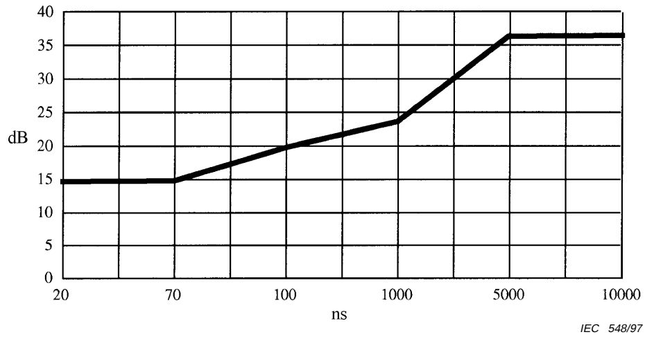
Figure B.1 – Exemple de rapport signal à écho acceptable en D2-MAC/paquet en FM
