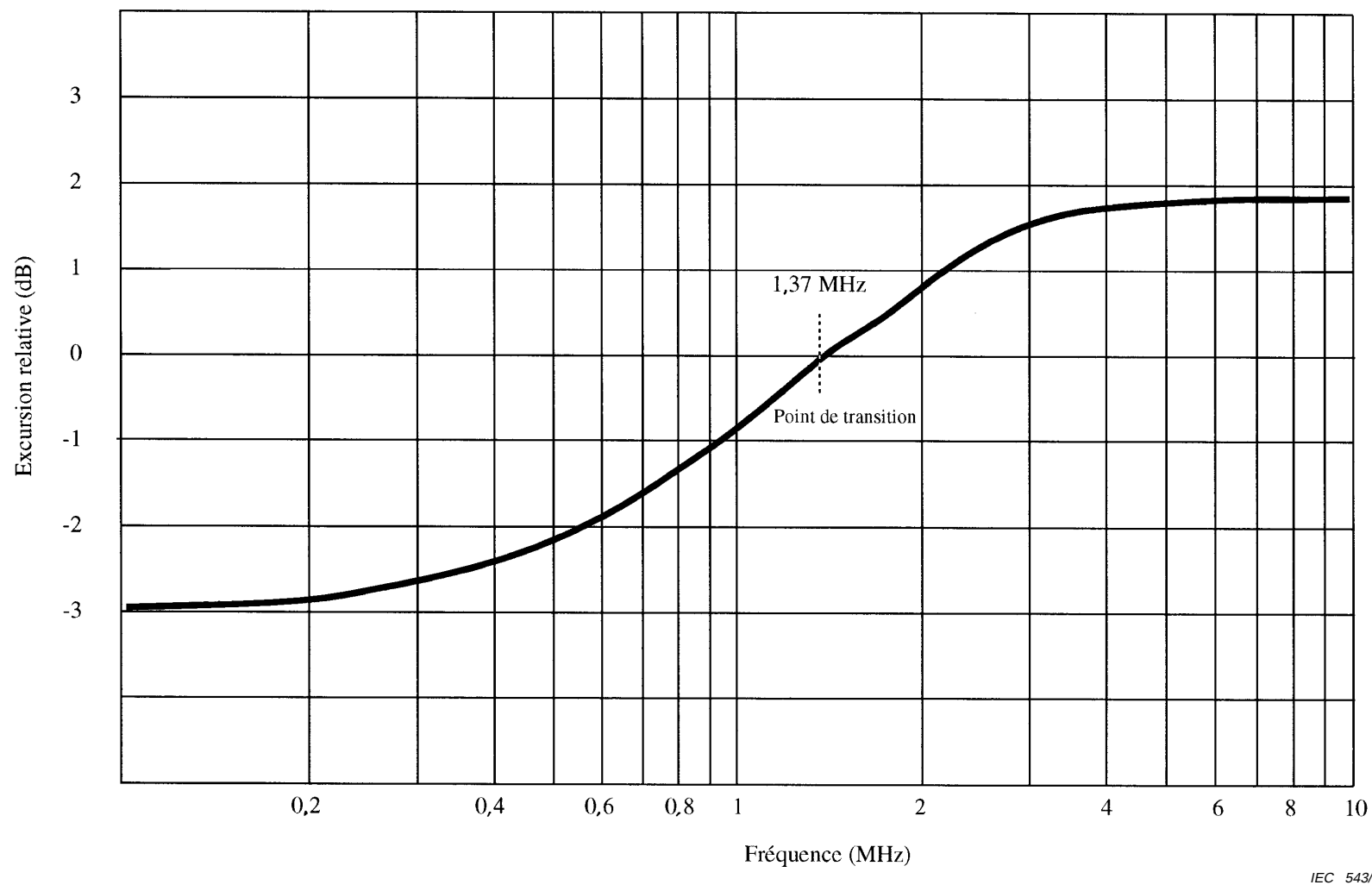
Figure A.1 – Préaccentuation pour le D2-MAC/paquet
