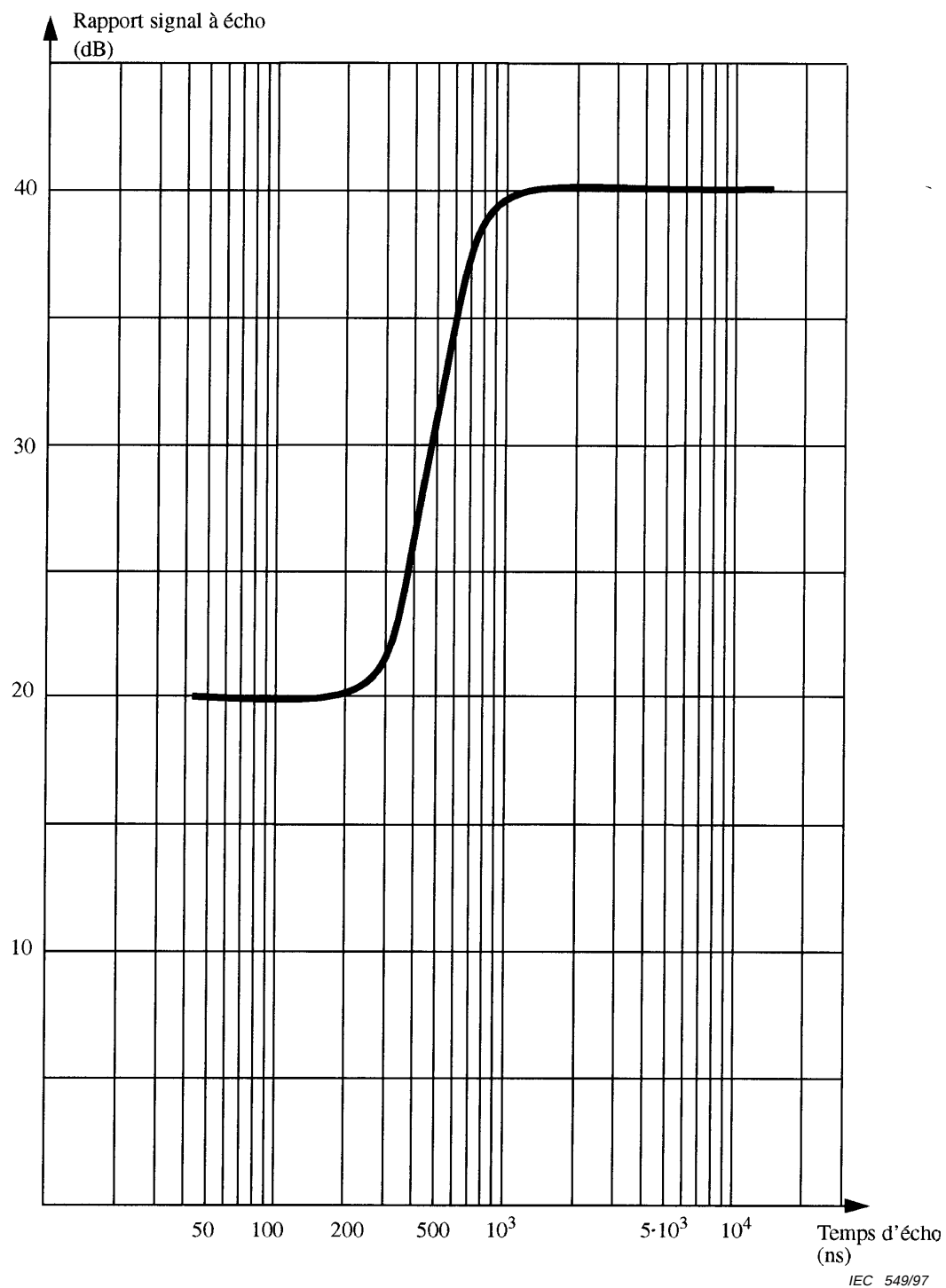
Figure B.2 – Exemple de rapport signal à écho acceptable en D2-MAC/paquet MA-BLR
