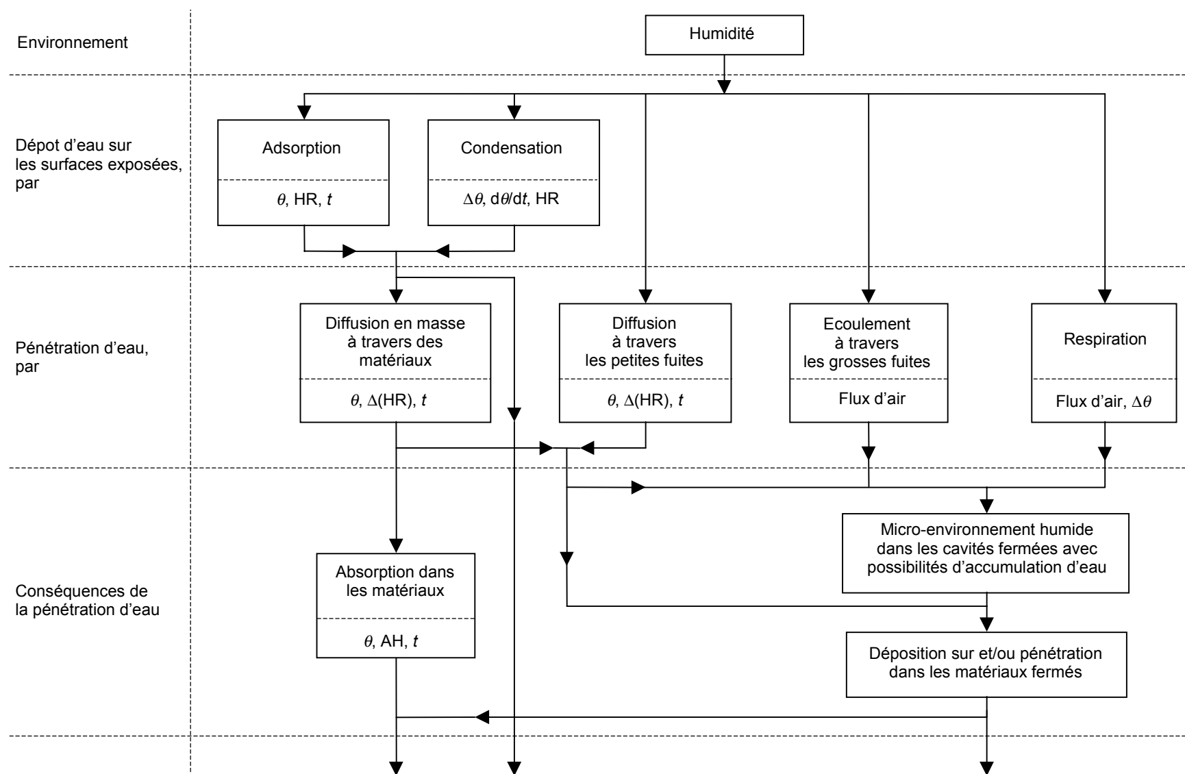
Figure A.1 – Phénomènes physiques intervenant dans les essais d'humidité
