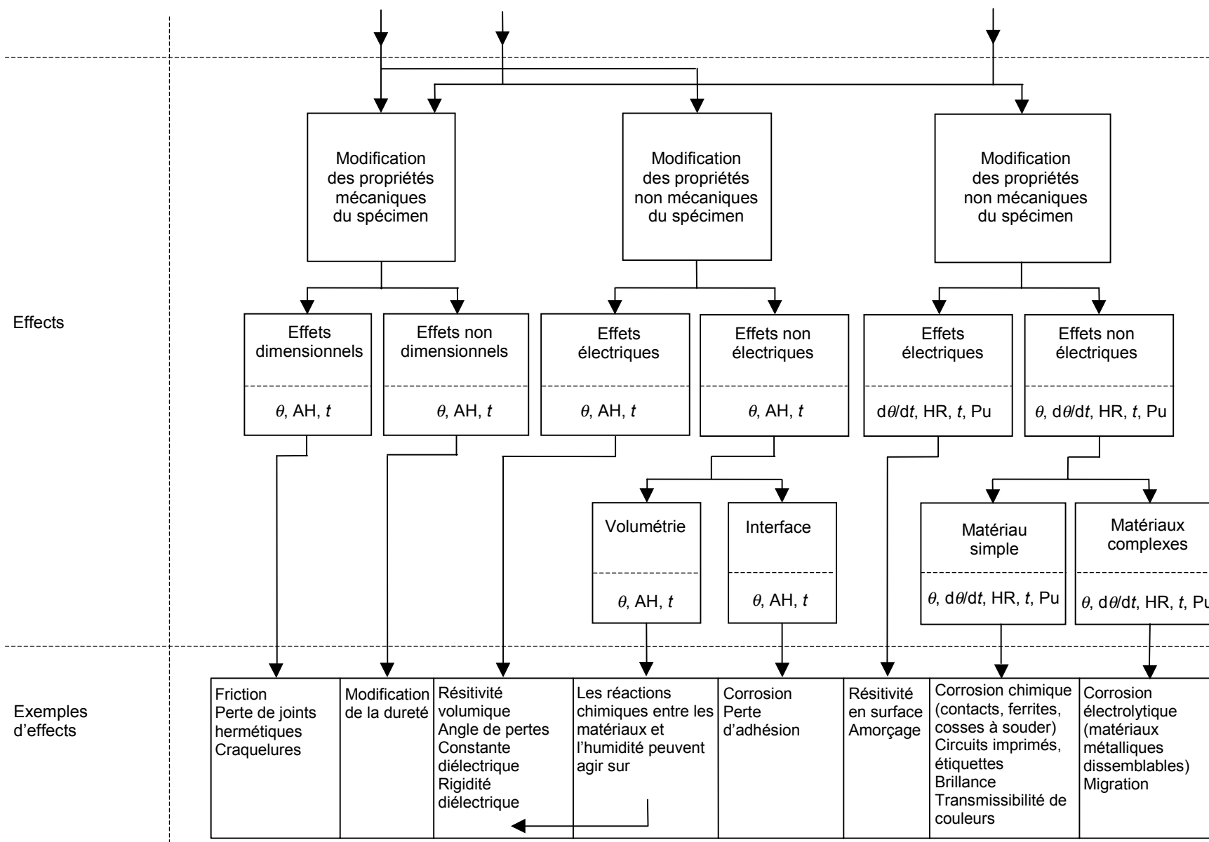
Figure A.1 – Phénomènes physiques intervenant dans les essais d'humidité (suite)
