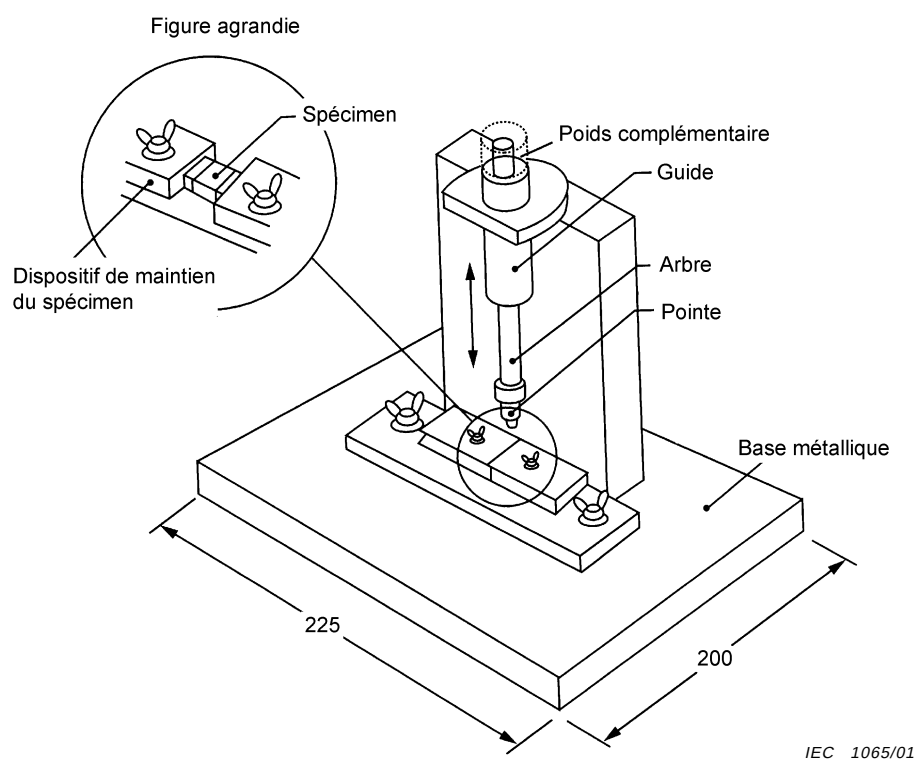
Figure 5 – Exemple d'équipement d'essai de chocs par impact
