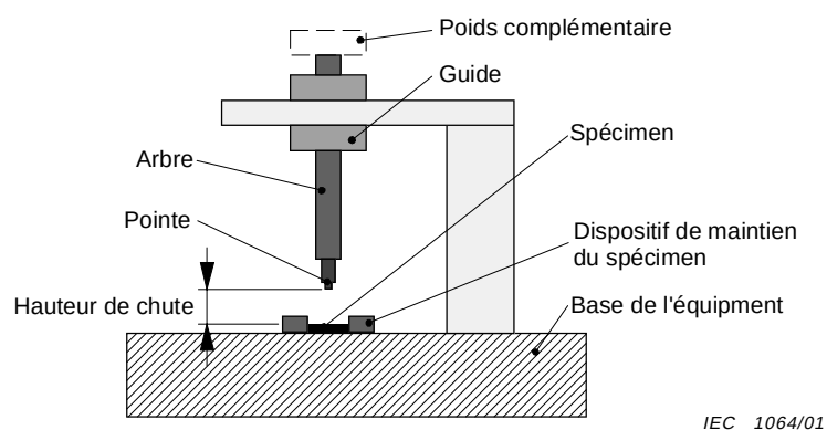
Figure 4 – Principe de l'équipement d'essai
