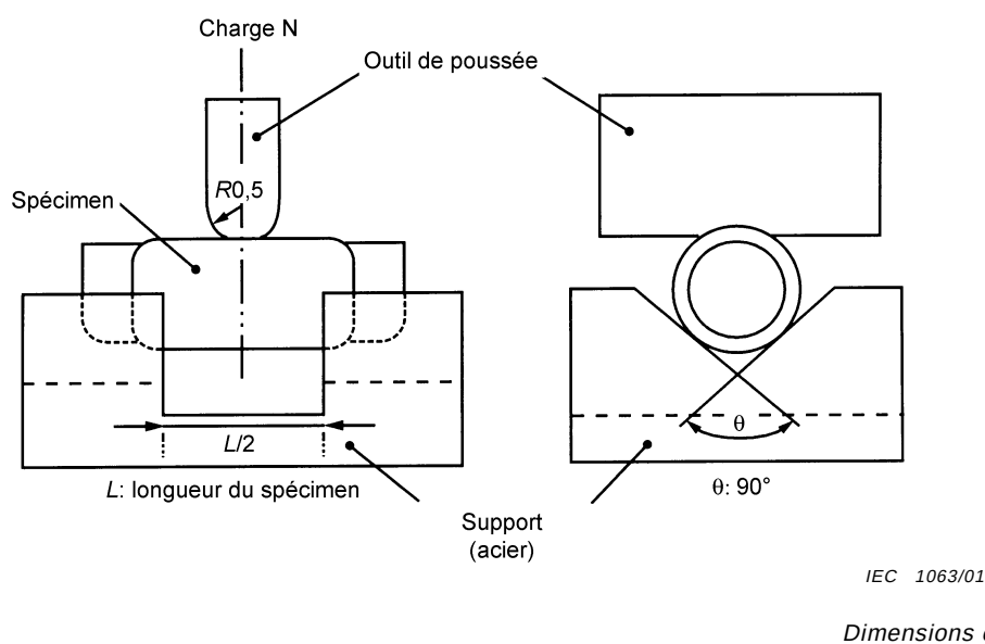
Figure 3 – Exemple d'essai de résistance du corps (pour condensateurs pastilles cylindriques en céramique)
