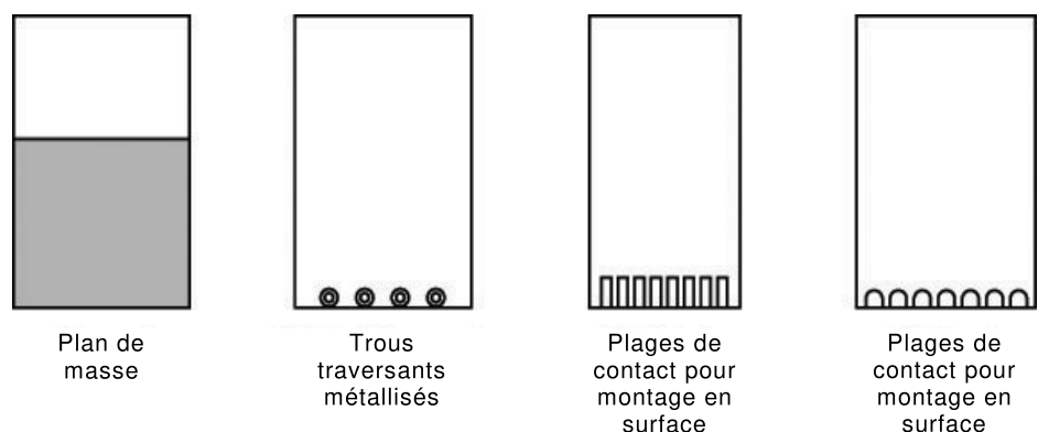
Figure 5 – Spécimens d'essai de balance de mouillage suggérés et immersion dans la brasure
