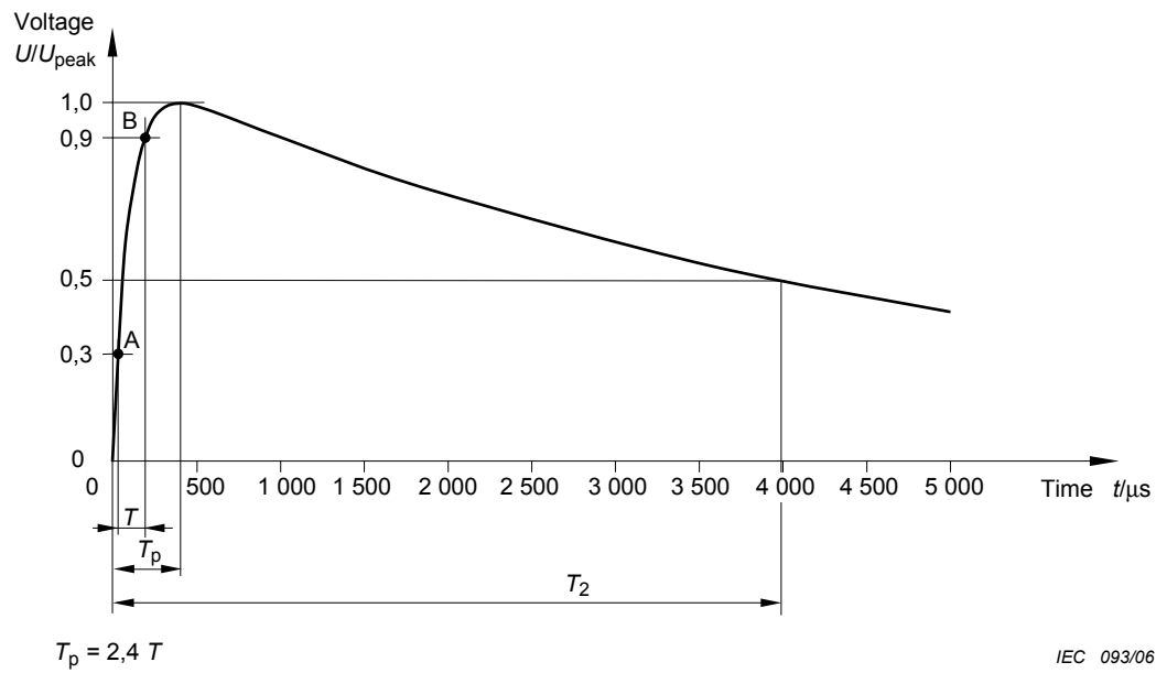
b) T_p/T_2 = 400/4\,000\ \mu\text{s}
