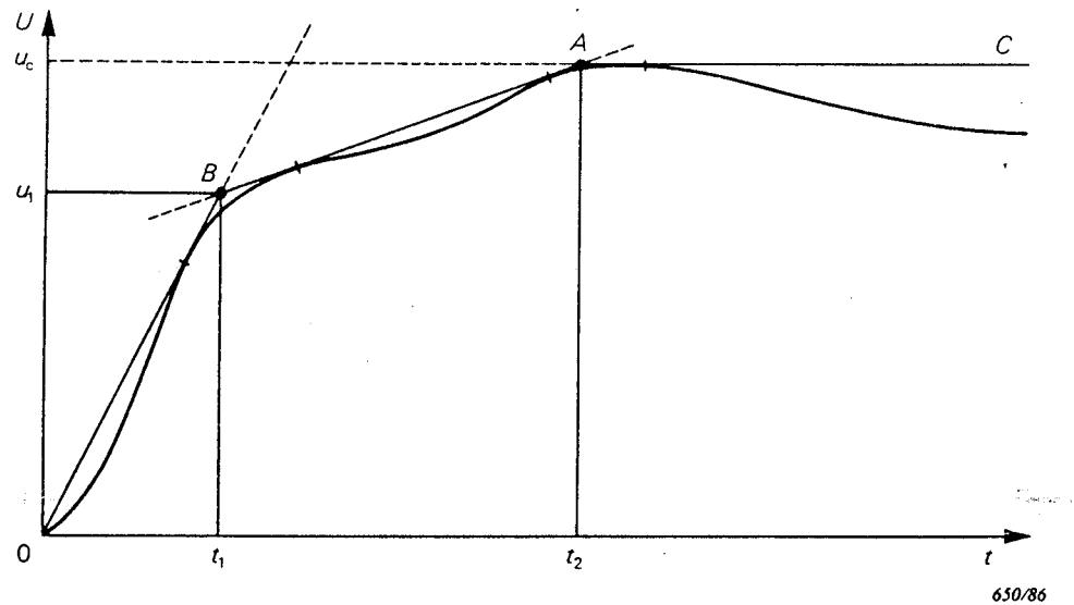
FIG. FF1. — Représentation par quatre paramètres d'une tension transitoire de rétablissement présumée d'un circuit. Cas du paragraphe FF2.3.1 de l'annexe FF.
