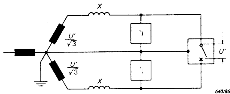
FIG. 30. — Circuit d'essai avec deux tensions décalées de 120 degrés électriques pour les essais en discordance de phases. Test circuit for out-of-phase tests using two voltages separated by 120 electrical degrees.
