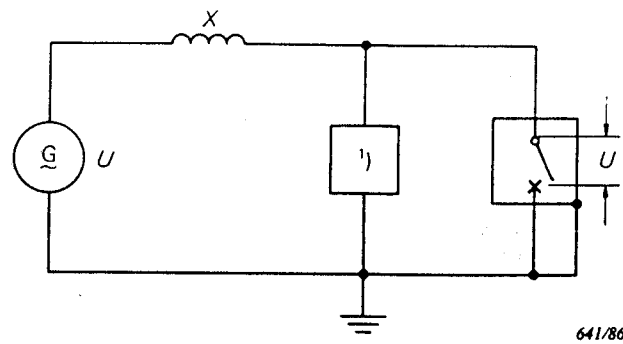
Fig. 31. — Circuit d'essai avec une borne du disjoncteur à la terre pour les essais en discordance de phases (sous réserve de l'accord du constructeur).
