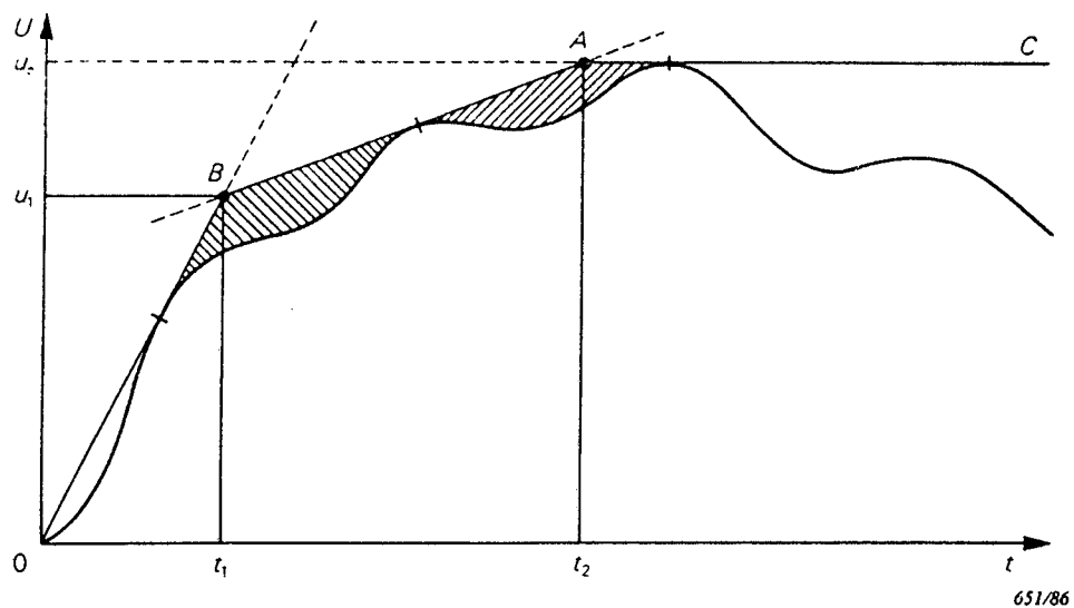
FIG. FF2. — Représentation par quatre paramètres d'une tension transitoire de rétablissement présumée d'un circuit. Cas du paragraphe FF2.3.2 de l'annexe FF.
