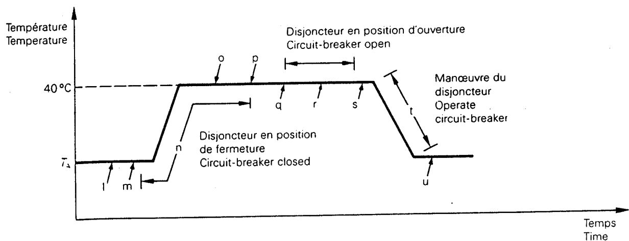
b) Essai à haute température High temperature test
