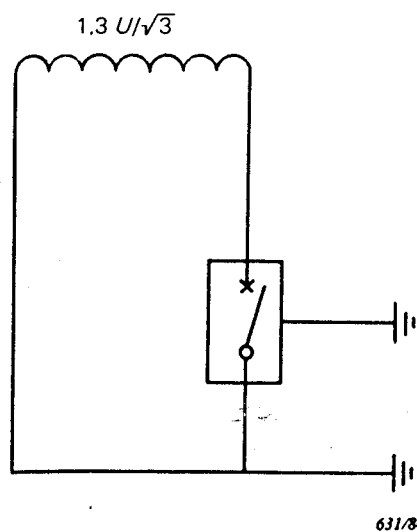
FIG. 22a. — Circuit préféré. Preferred circuit.
