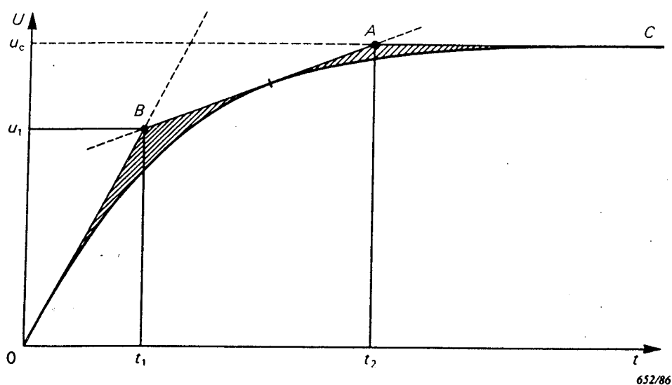
Fig. FF3. — Représentation par quatre paramètres d'une tension transitoire de rétablissement présumée d'un circuit. Cas du paragraphe FF2.3.3 a) de l'annexe FF. Representation by four parameters of a prospective transient recovery voltage of a circuit. Case of Sub-clause FF2.3.3 a) of Appendix FF.
