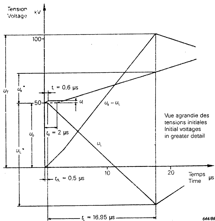
FIG. AA1. — Construction d'une TTR pour défaut proche en ligne. Construction of TRV for short-line fault.
