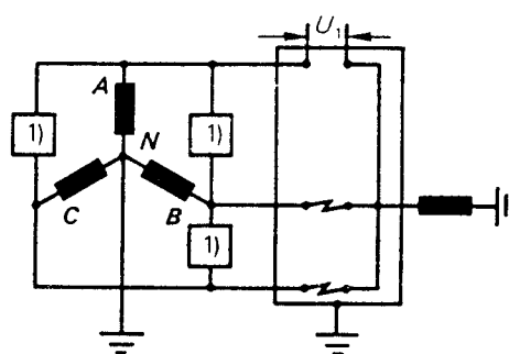
FIG. 20b. — Circuit utilisé en variante. Alternative circuit.
