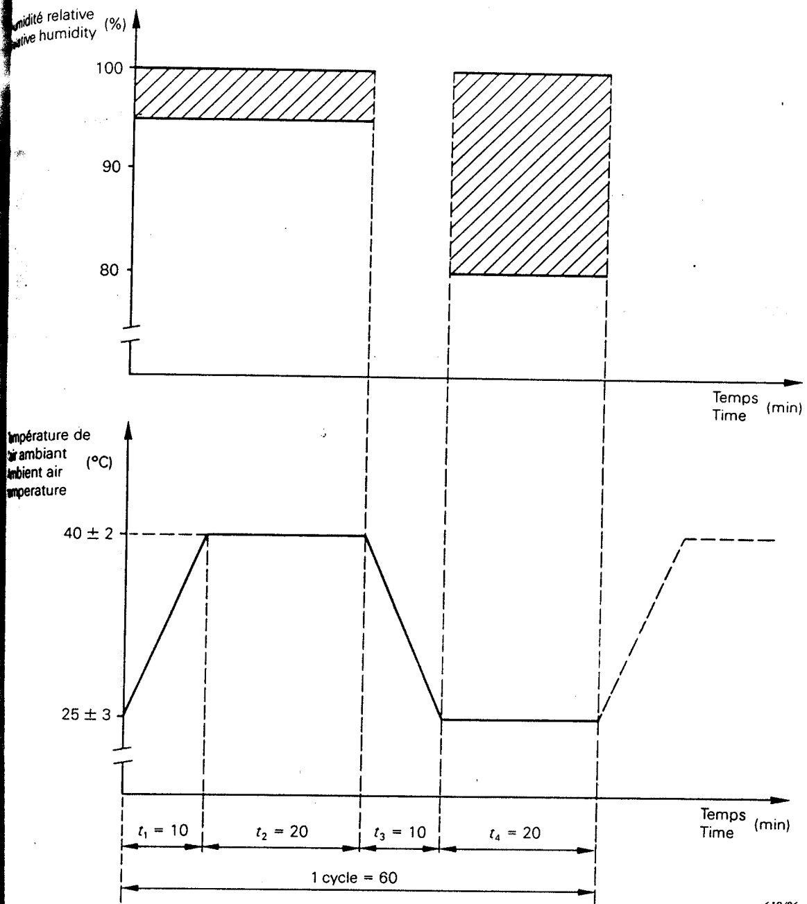
FIG. 16. — Essai à l'humidité. Humidity test.
