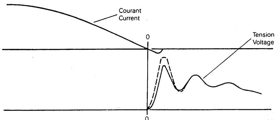
FIG. GG5. — Coupure avec courant post-arc. Breaking with post-arc current.
