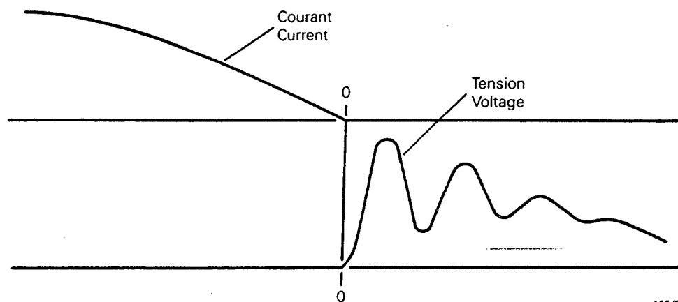
FIG. GG2. — TTR pour une coupure idéale. TRV in case of ideal breaking.
