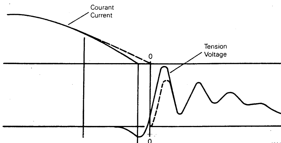
FIG. GG3. — Coupure avec présence d'une tension d'arc. Breaking with arc-voltage present.
