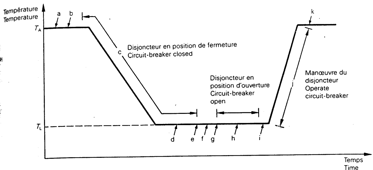
a) Essai à basse température Low temperature test
