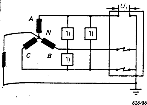
FIG. 20a. — Circuit préféré. Preferred circuit.
