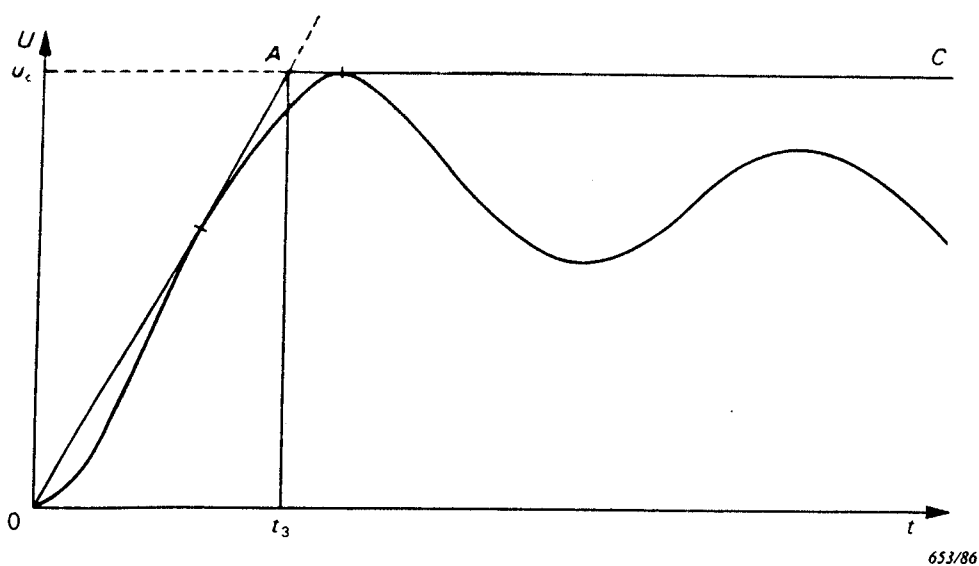
Fig. FF4. — Représentation par deux paramètres d'une tension transitoire de rétablissement présumée d'un circuit. Cas du paragraphe FF2.3.3 b) de l'annexe FF. Representation by two parameters of a prospective transient recovery voltage of a circuit. Case of Sub-clause 2.3.3 b) of Appendix FF.
