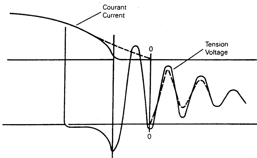
FIG. GG4. — Coupure avec arrachement prononcé du courant. Breaking with pronounced premature current-zero.
