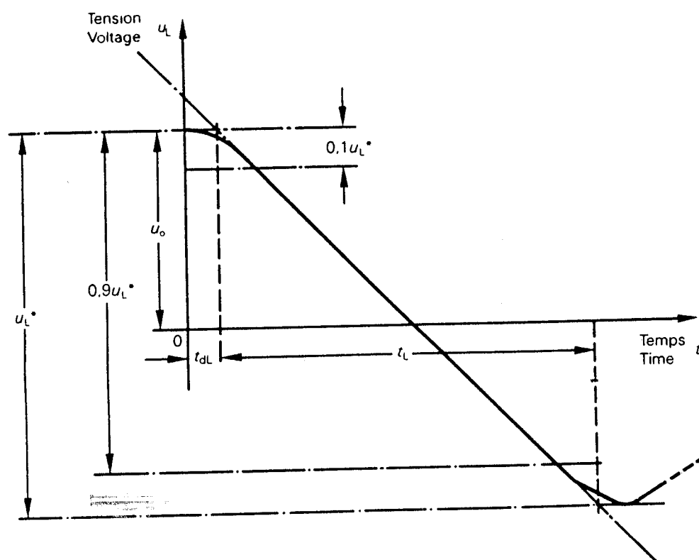
FIG. 14. — Exemple d'une tension transitoire côté ligne avec un retard et une crête arrondie montrant la construction à effectuer pour obtenir les valeurs u_L^* , t_L et t_{dL} . Example of a line-side transient voltage with time delay and rounded crest showing construction to derive the values u_L^* , t_L and t_{dL} .
