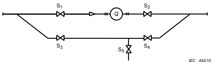
Figure 5 – Tuyauterie de dérivation
