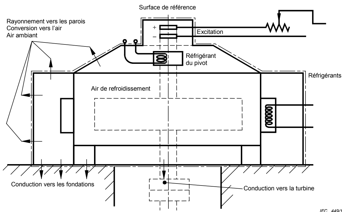
Figure 2 – Surface de référence
