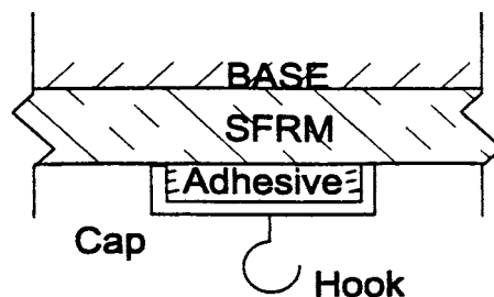
FIG. 2 In-Place Apparatus
