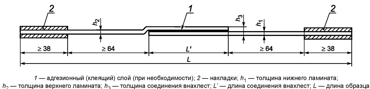
Рисунок 2 — Размеры односрезных образцов изготовленного способом мокрого формования FRP
