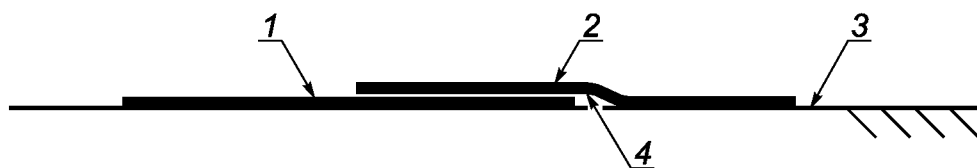
1 — нижний слоистый материал; 2 — верхний слоистый материал; 3 — поверхность технологической оснастки; 4 — изгиб в верхнем слоистом материале для изготовленной методом мокрого формования усиленной волокнами пластмассы (FRP)
