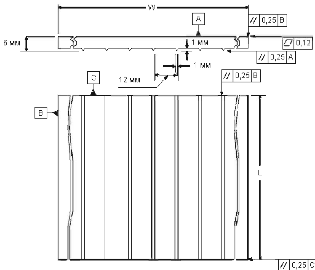
Рисунок 1 — Зубчатая пластина
