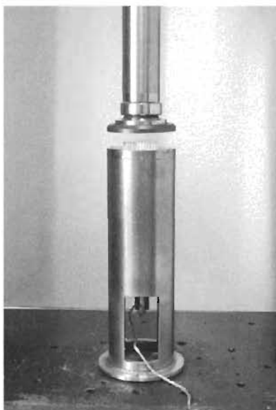
Рисунок 1 — Плита пресса с датчиком и регулировкой стержня
