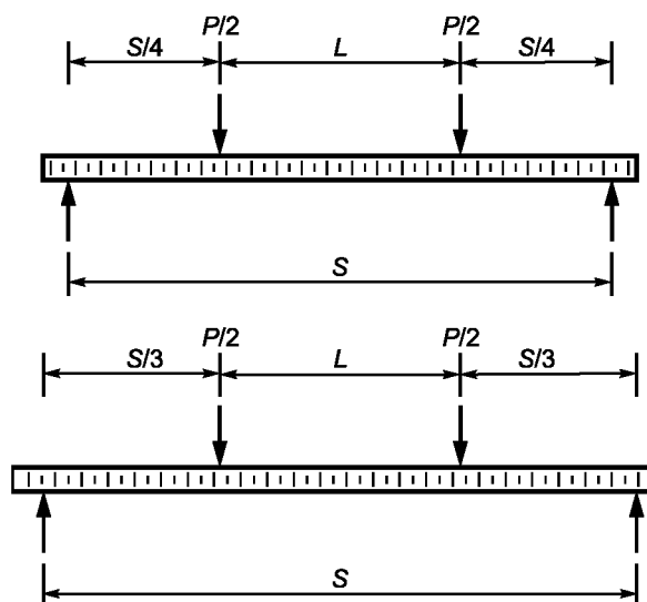
(с) четырехточечное нагружение (С393/С393М нестандартная схема)
