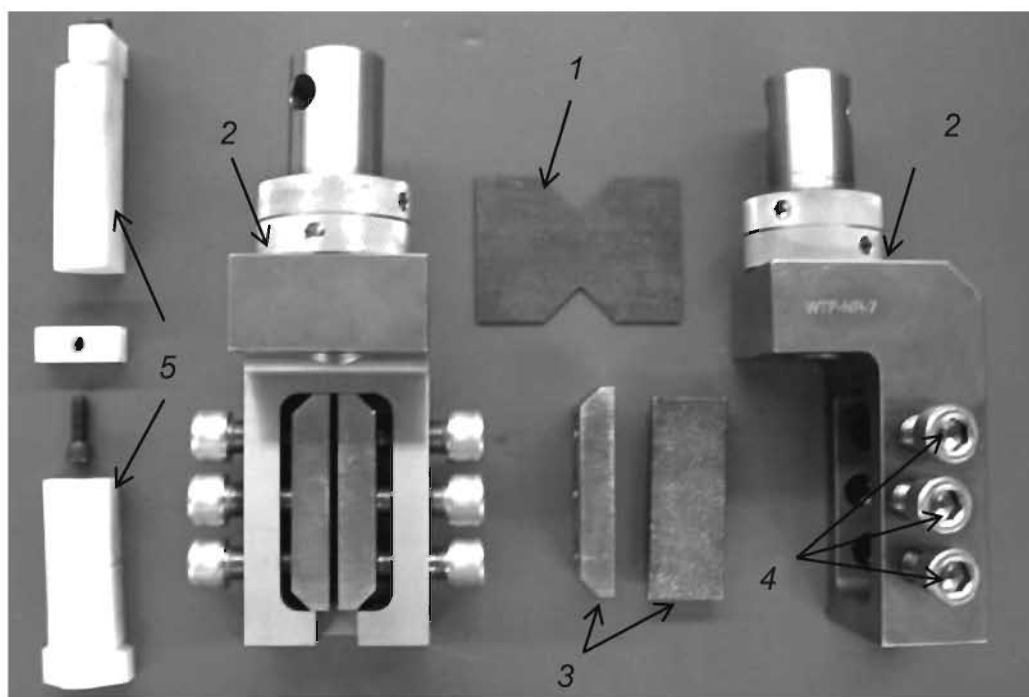
Рисунок 2 — Собранное приспособление для испытаний на сдвиг образца с V-образными надрезами
