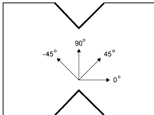
Рисунок 6 — Ориентация волокон в образце с V-образными надрезами
