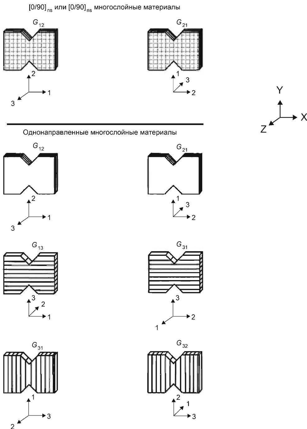
Рисунок 5 — Ориентация плоскостей в материале
