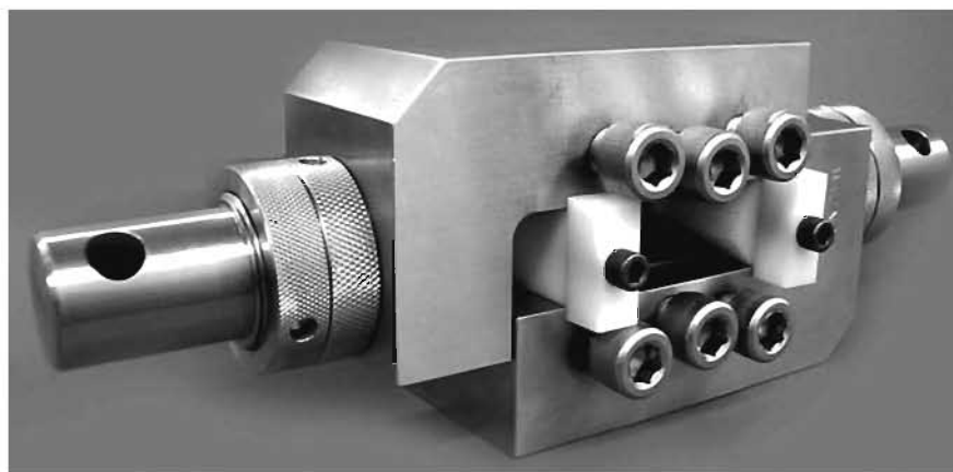
Рисунок 8 — Использование разделительных блоков для выравнивания половин приспособления
