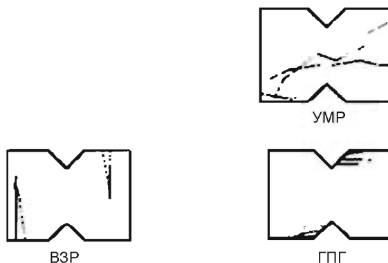
Некорректные типы разрушения
