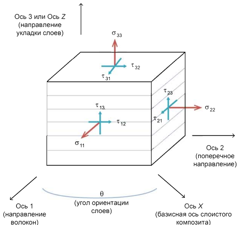
Рисунок 1 — Система координат материала
