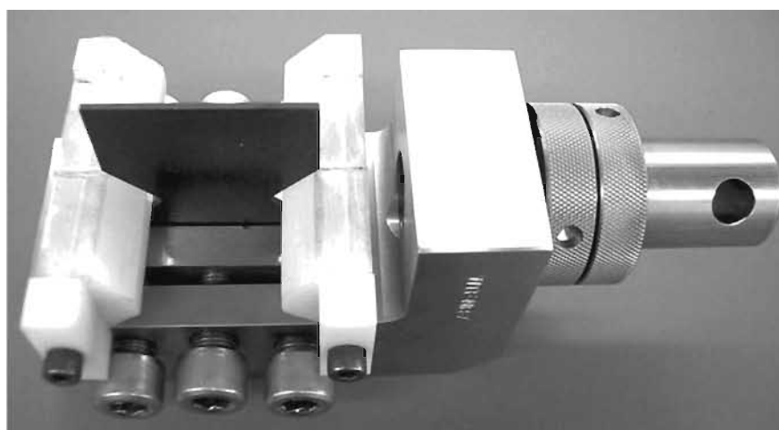
Рисунок 7 — Использование разделительных блоков для выравнивания образца
