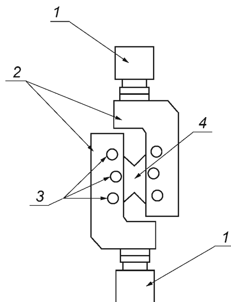
Рисунок 2 — Собранное приспособление для испытаний на сдвиг образца с V-образными надрезами
