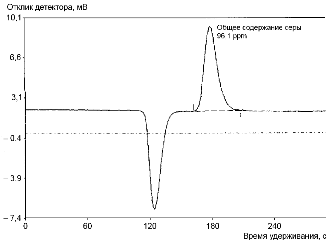
Рисунок 1 – Типовая хроматограмма
