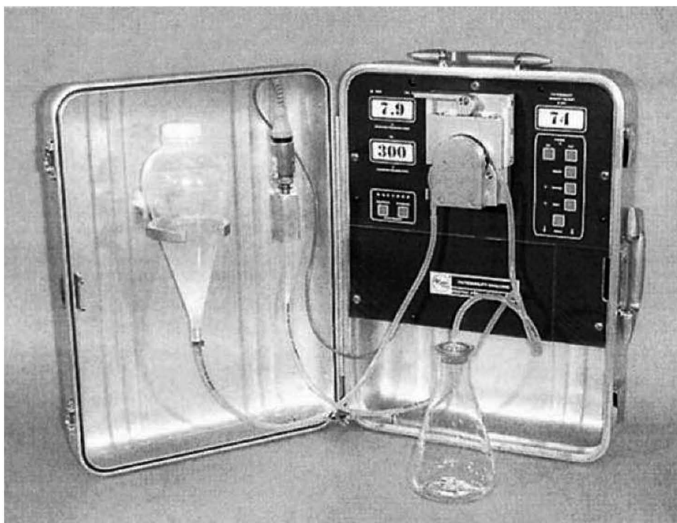
Рисунок 2 — Микроанализатор для определения фильтруемости
