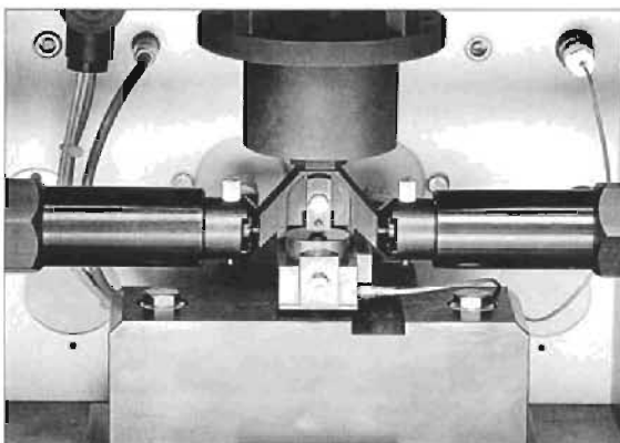
Рисунок 2 – Испытательная камера
