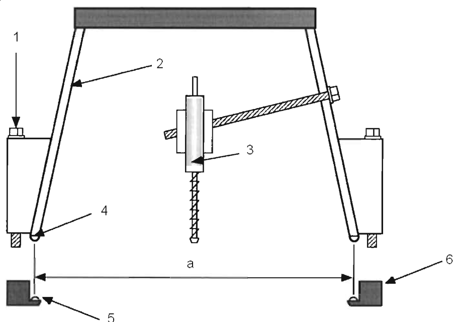
a — расстояние между опорными подшипниками; 1 — болты крепления, соединяющие верхнюю и нижнюю части приспособления для испытания; 2 — верхняя часть приспособления для испытания; 3 — датчик перемещения; 4, 5 — опорные подшипники; 6 — нижняя часть приспособления для испытания
