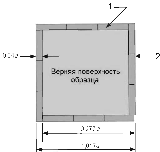
1 — металлические пластины; 2 — грани образцов, подверженные разрушению
