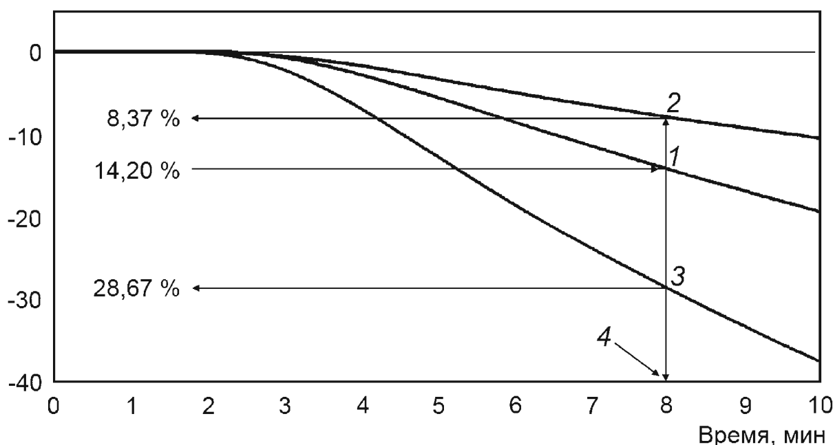
Рисунок 4 – Определение стандартного времени методом Ноак и потери от испарения испытуемых масел
