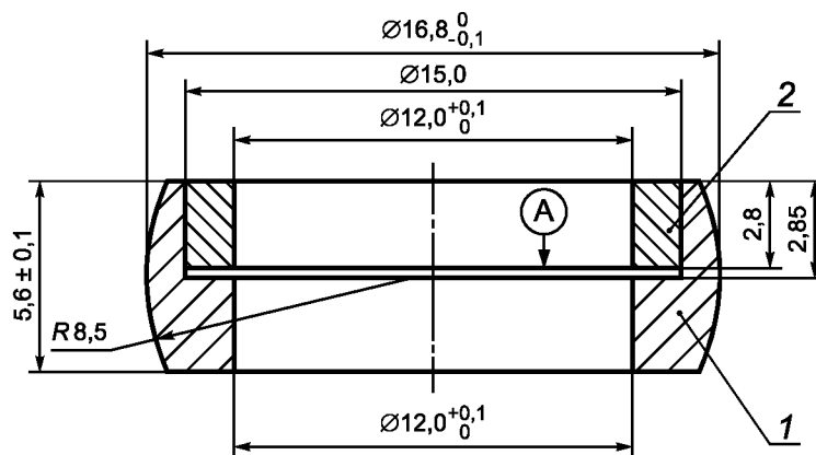
Рисунок 8 — Латунный держатель фильтра
