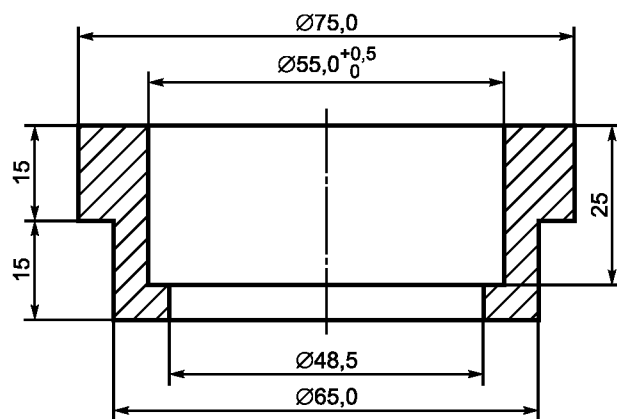
Рисунок 4 — Стопорное кольцо
