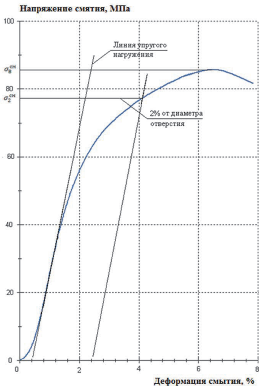
Рисунок 6 — Диаграмма смятия
