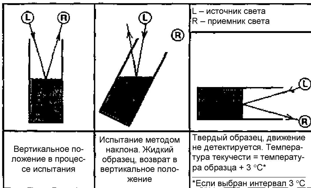
Рисунок 1 – Оптическая система детектирования
