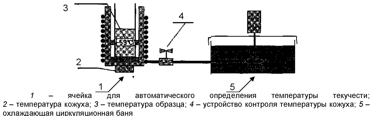
Рисунок 2 – Схема испытательной ячейки для определения температуры текучести и охлаждающей циркуляционной бани
