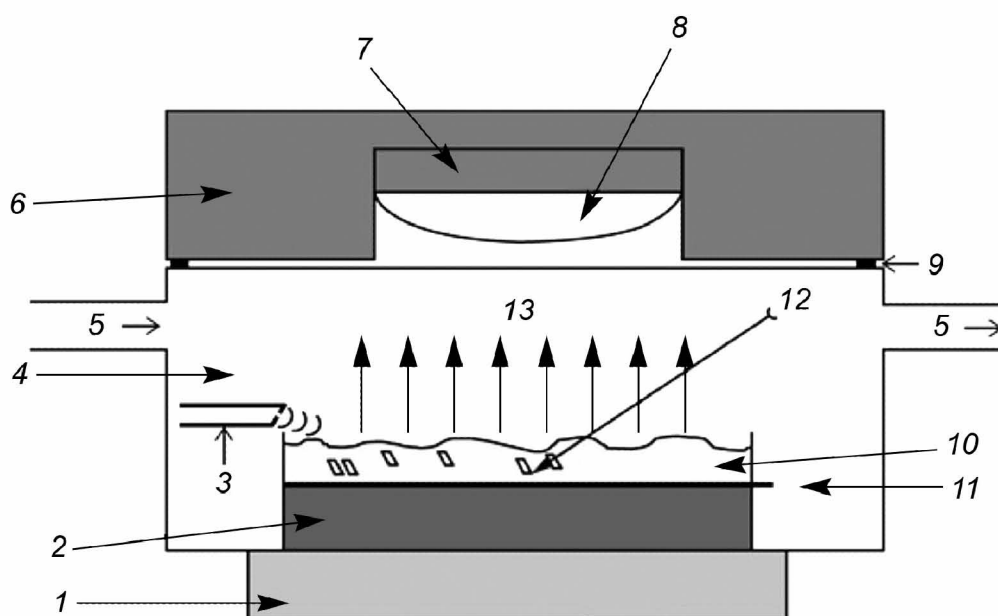
Рисунок А1.1 — Схематическое изображение испытательной ячейки
