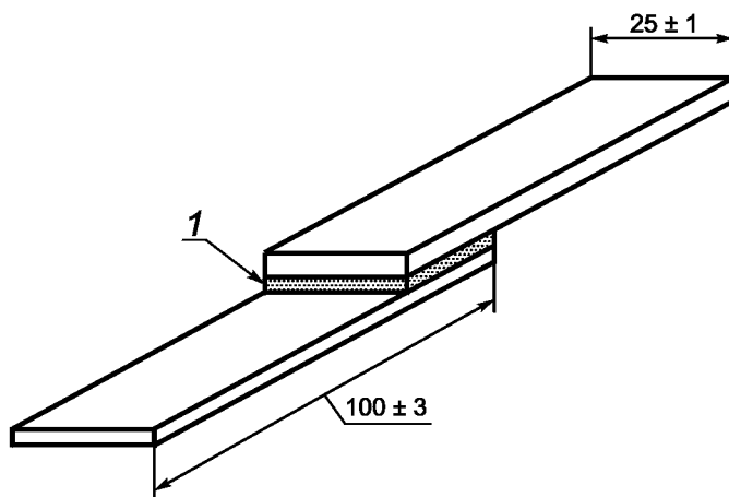
Рисунок 1 — Соединение внахлест
