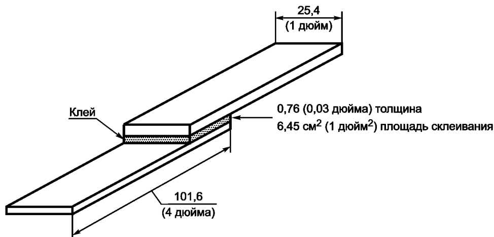
Рисунок 1 — Соединение внахлест
