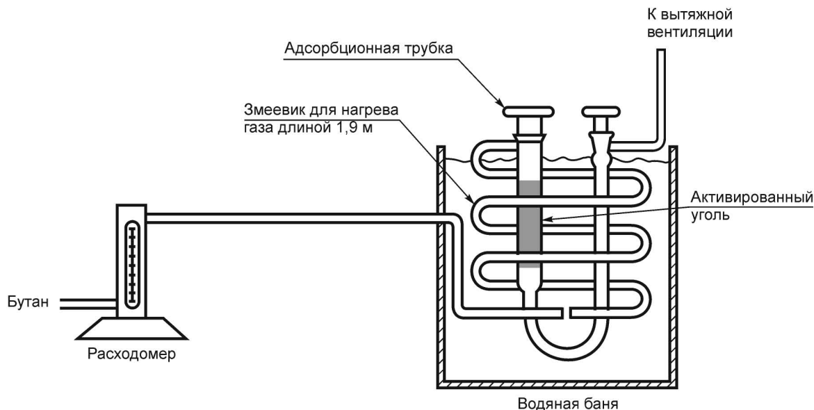
Рисунок 3 — Схема установки для определения активности по бутану
