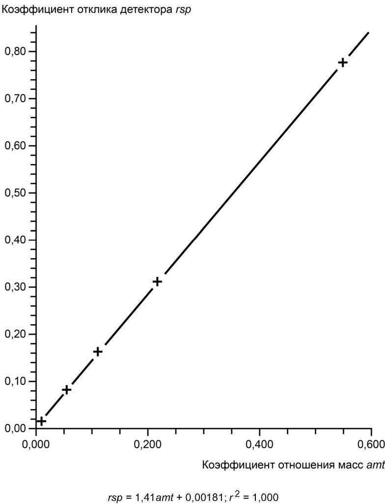
Рисунок 3 — Типовая калибровочная кривая для бензола
