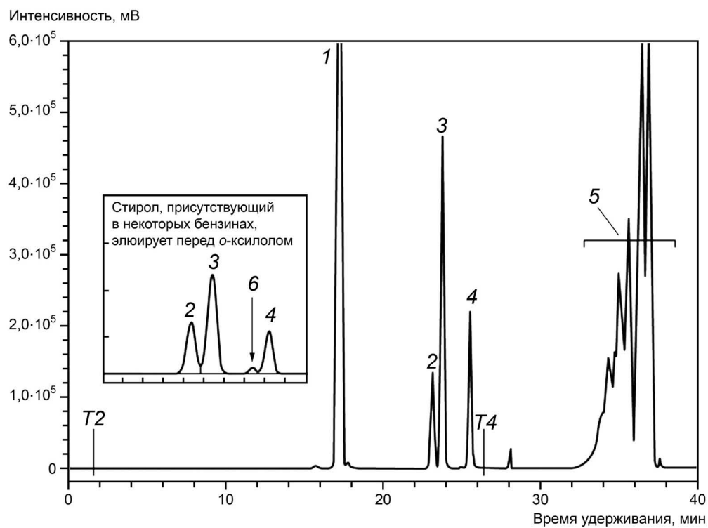
1 — 2-гексанон (внутренний стандарт); 2 — этилбензол; 3 — p/m -ксилол; 4 — o -ксилол; 5 — C_{9+} ароматические углеводороды; 6 — стирол
