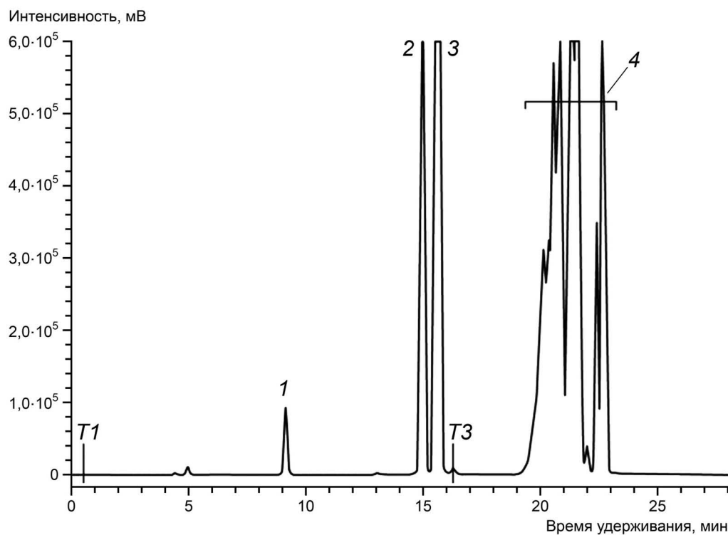
1 — бензол; 2 — толуол; 3 — 2-гексанон (внутренний стандарт); 4 — пик обратной промывки (ароматические компоненты C_{8+} и C_{9+} неароматические углеводороды)
