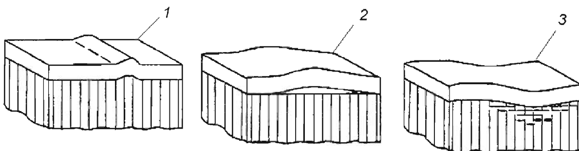
1 — образец разрушения, характер разрушения ВГМ; 2 — образец разрушения, характер разрушения ДГМ; 3 — образец разрушения, характер разрушения СГМ
