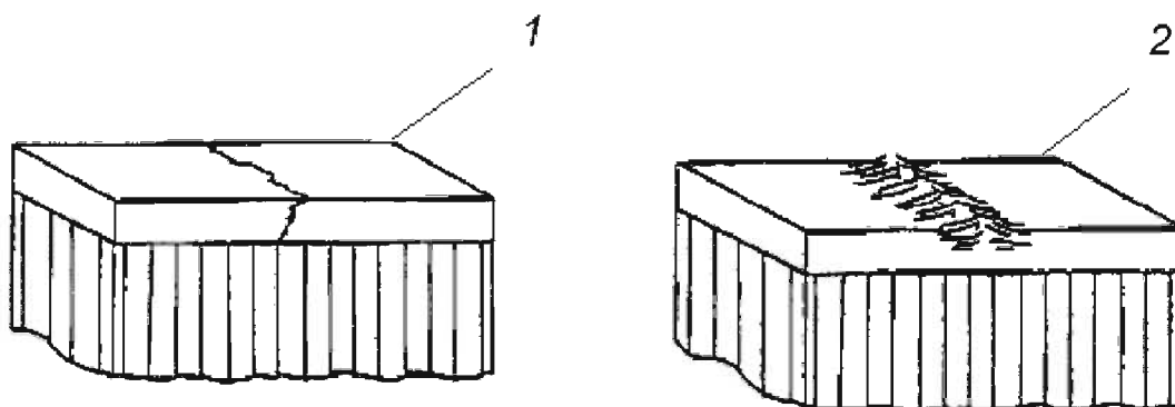
1 — образец разрушения, характер разрушения НГМ; 2 — образец разрушения, характер разрушения ФГМ
