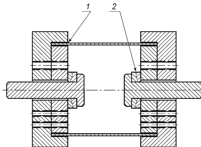
1 — клей; 2 — сферические шайбы для самоцентрирования
