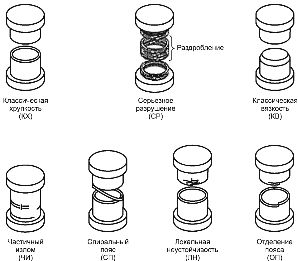
Рисунок 4 — Виды разрушения образцов кольцевой намотки при сжатии
