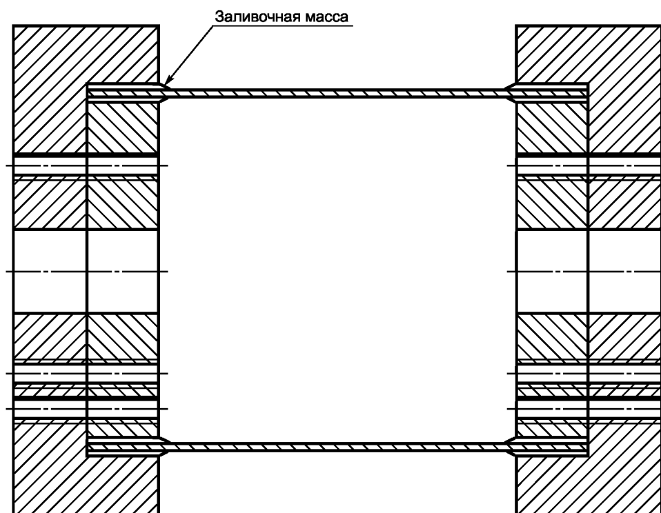
Рисунок 3 — Образец ПКМ, закрепленный в приспособлении для сжатия
