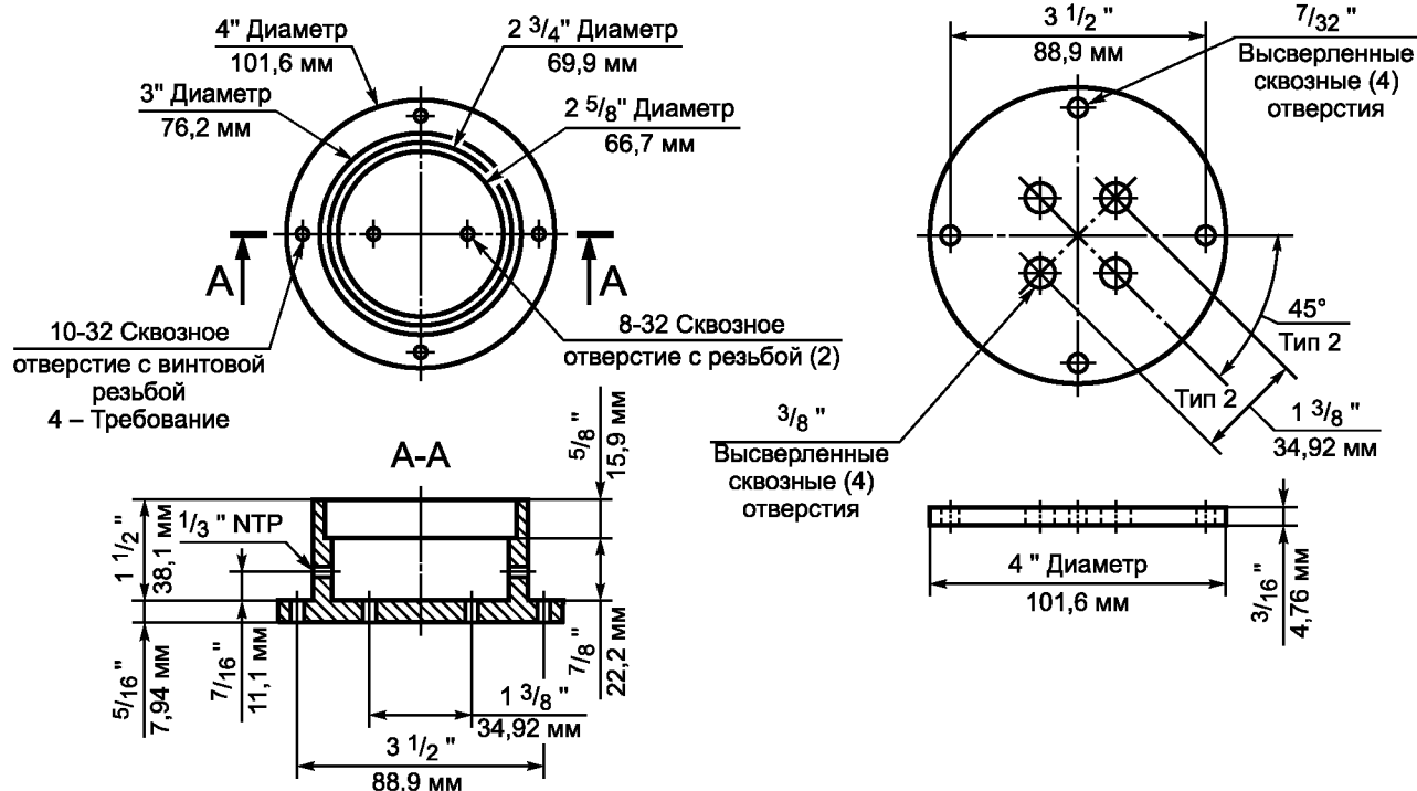
Вытяжная секция "AA" ~ (1) требование – алюминий
