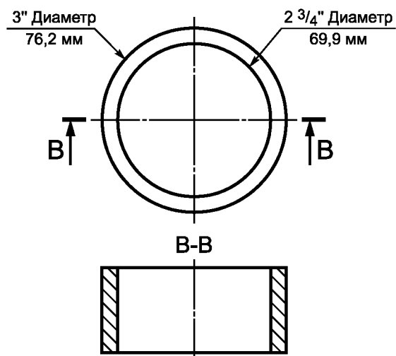
Прибордержатель и разделительная секция "BB" ~ (2) требование – алюминий
