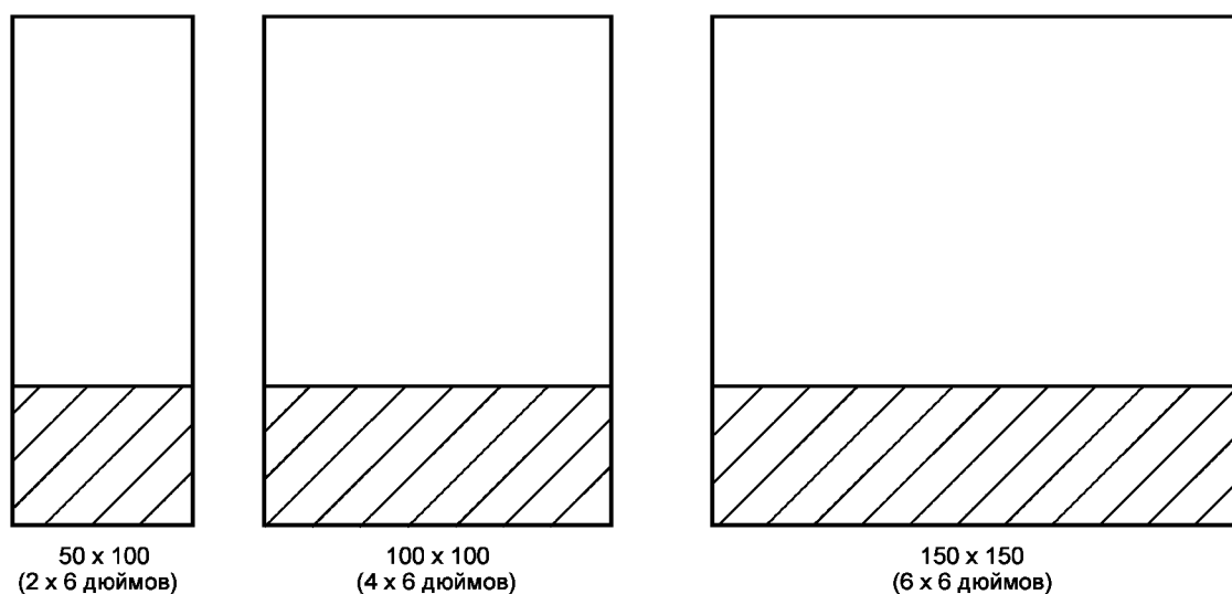
Рисунок X1.2 — Размеры образцов
