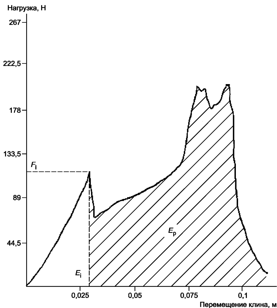
Рисунок 1 — График зависимости изменения нагрузки от перемещения клина
