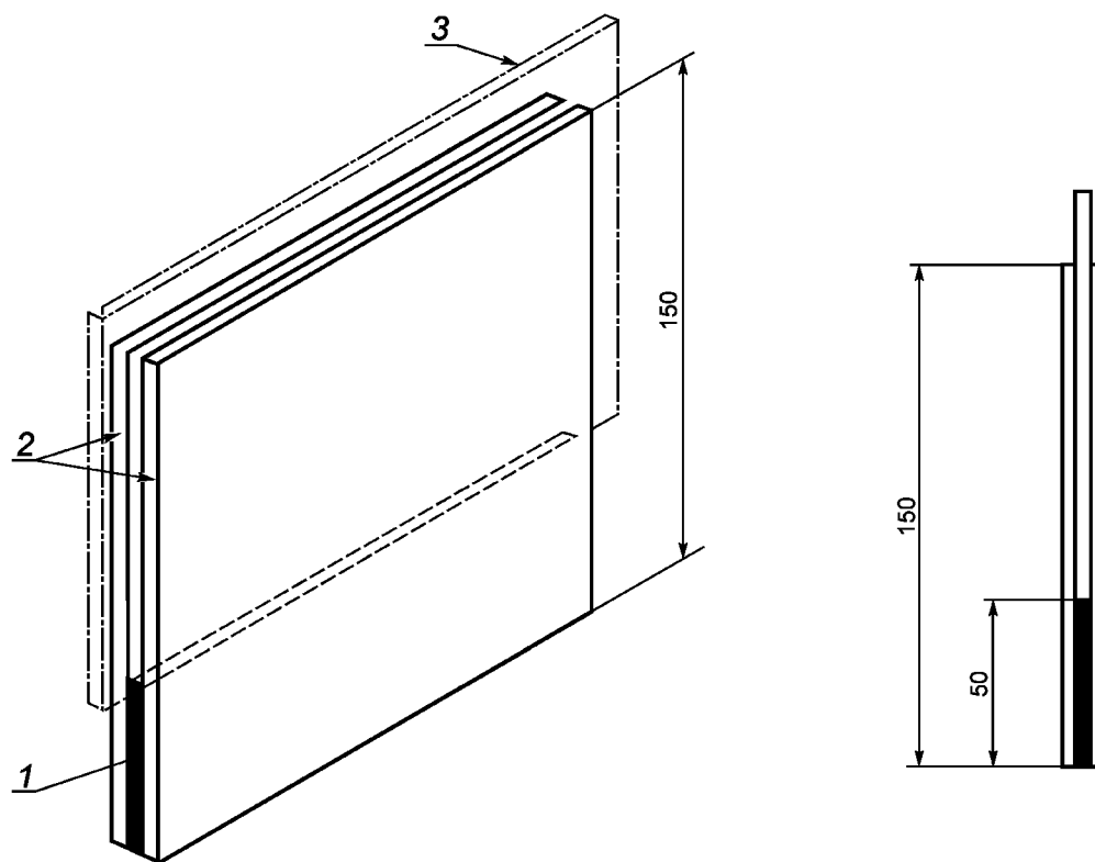
1 — клей; 2 — подложки; 3 — съемная прокладка
