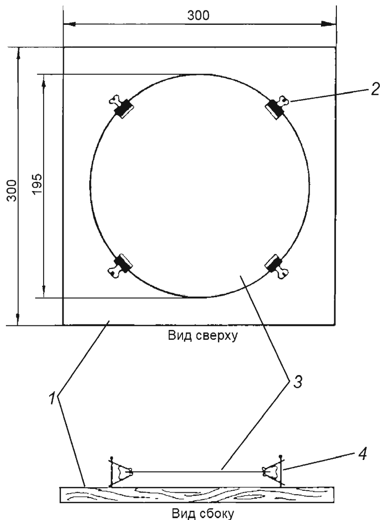
Рисунок 1 — Держатель бумаги для испытания
