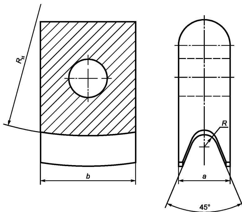
Рисунок 1 — Пуансон для испытания образцов круглого сечения
