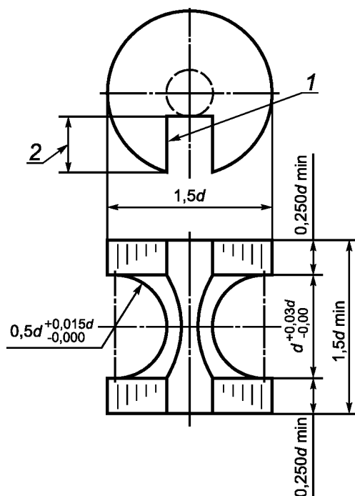
1 — шпоночная канавка; 2 — глубина до нижней границы радиуса; d — диаметр образца
