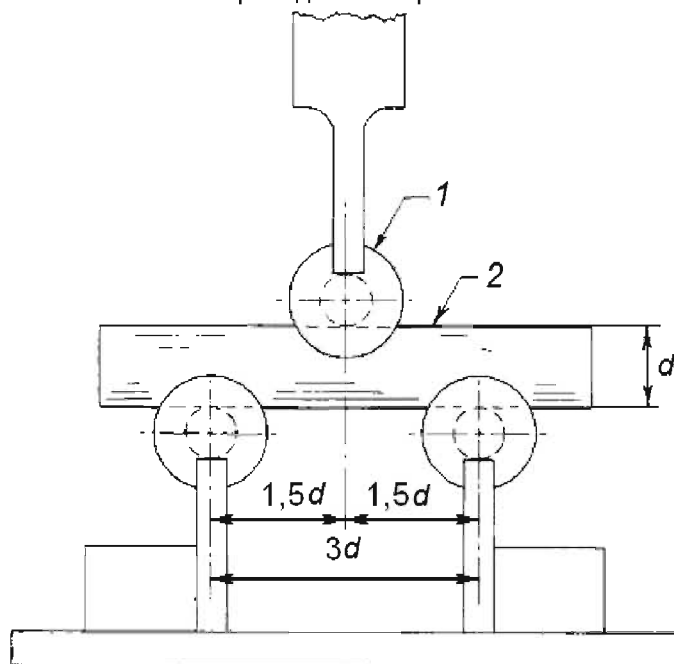
1 — пуансон; 2 — образец; d — диаметр образца
