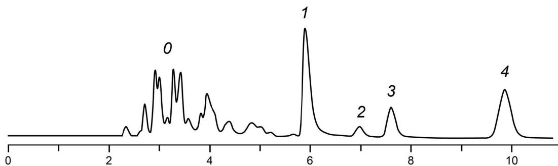
Рисунок X1.5 — Пример хроматограммы (газ-носитель — гелий)
