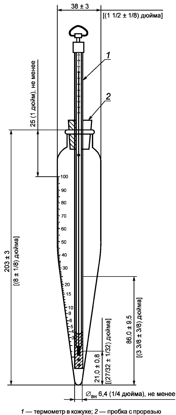
Рисунок 1 — Пробирка
