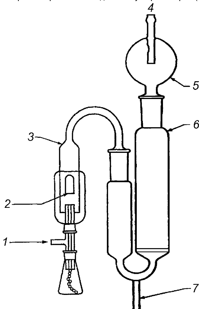
Рисунок 1 – Схема лампового узла
