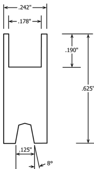
FIG. 3 Anode Cap
