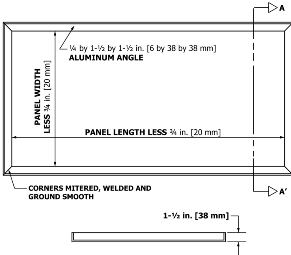
SECTION A-A' FIG. 1 Sag Test Frame
