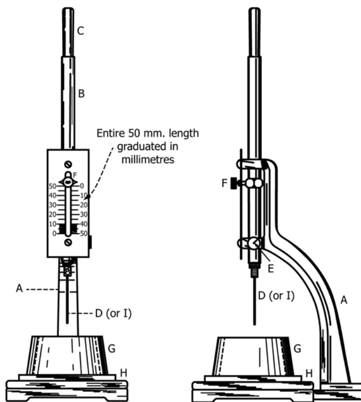
FIG. 1 Vicat Apparatus
