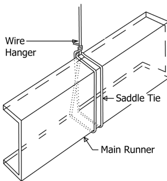
FIG. 3 Saddle-Tie
